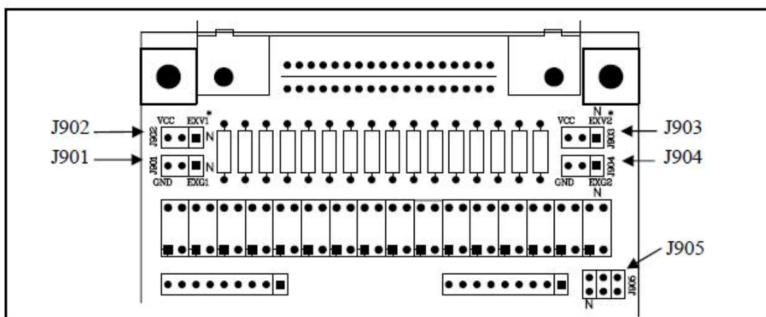
图 8-7 跳线在 HANDLER 接口板上的位置
