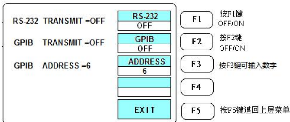
图4-21 总线设置菜单
