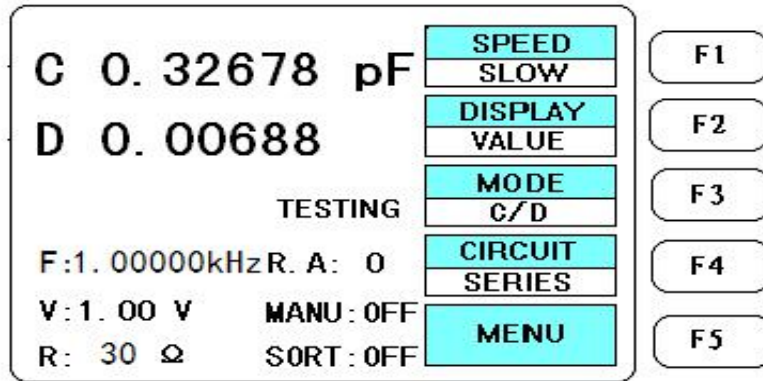
图4-1 测量状态显示图
