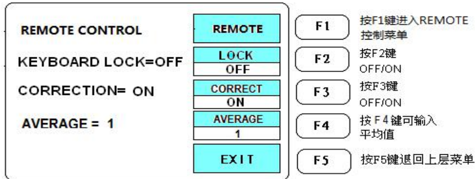
图 4-20 有效设置设定菜单
