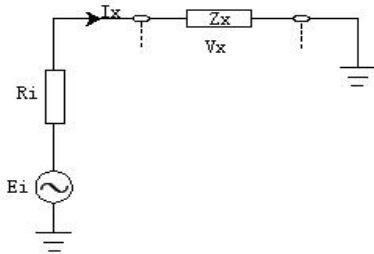
图 5-5 仪器信号源输出等效图
