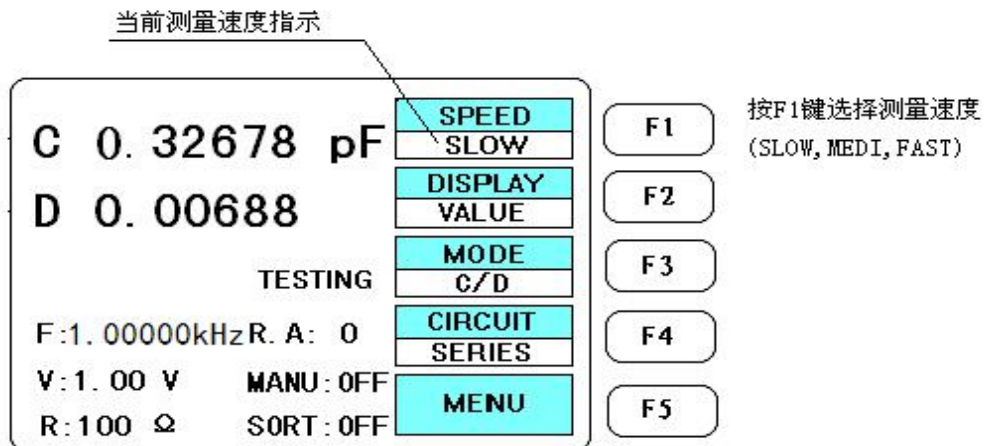
图 4-3 测量速度选择
