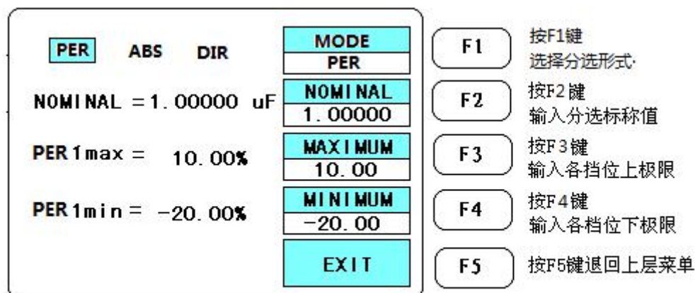
图 4-17 主参数 分选极值设定菜单
