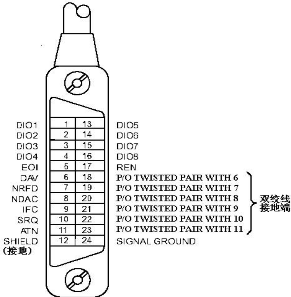
图 6-3 GPIB 接插件/管脚结构图
