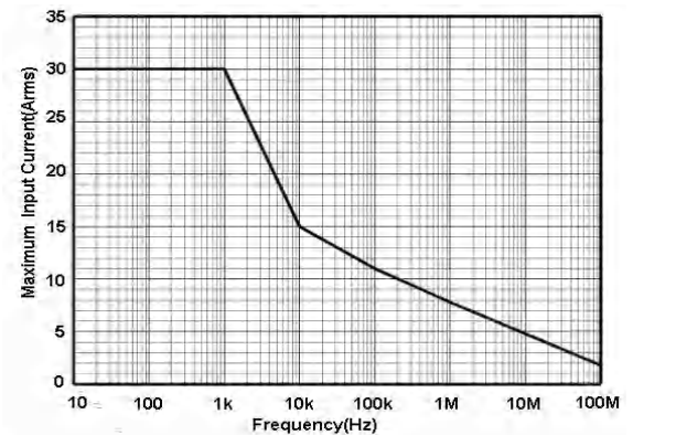
图 2.c HCP8030D 最大测量电流 VS 频率曲线
