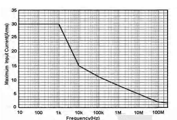
图 2.d HCP8030H 最大测量电流 VS 频率曲线
