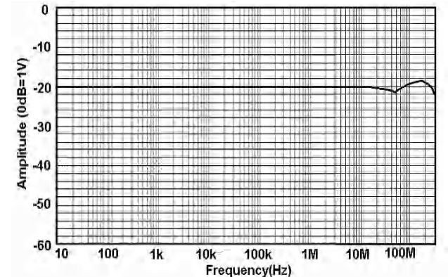
图 1.d HCP8030H 幅频曲线
