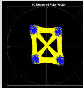
校准后的 AWGN 可仿真噪声环境。
