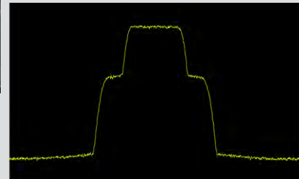
校准后的 AWGN 可仿真噪声环境。
