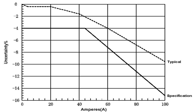
图 4 典型的 DC 线性度 (0.01V/A 档位)
