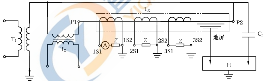
图 26 绝缘热稳定试验(线路 1)
