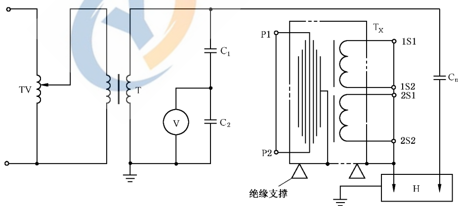
图 13 电容型互感器部分电容量和介质损耗因数测量(正接法)
