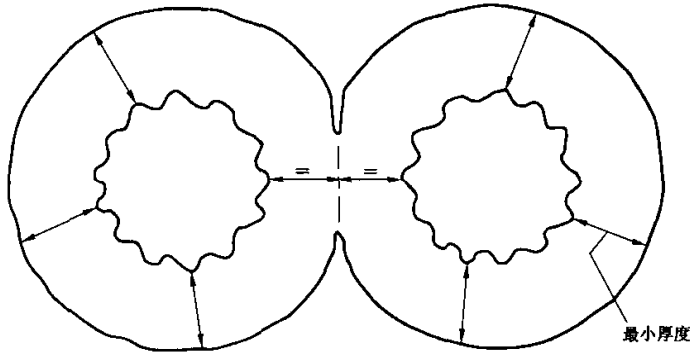
图 6 绝缘厚度测量(扁平双芯无护套软线)
