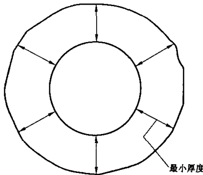
图 1 绝缘和护套厚度测量(圆形内表面)
