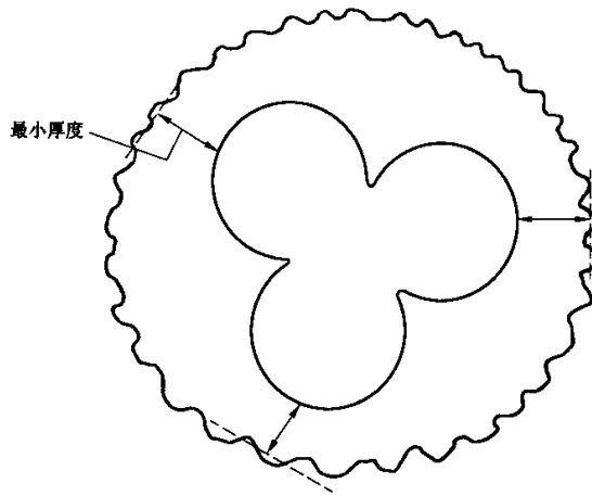
图 9 护套厚度测量(不规整外表面)
