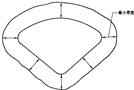
图 2 绝缘厚度测量(扇形导体)
