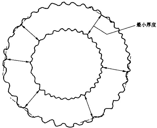
图 5 绝缘厚度测量(不规整外表面)
