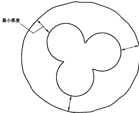
图 8 护套厚度测量(非圆形内表面)
