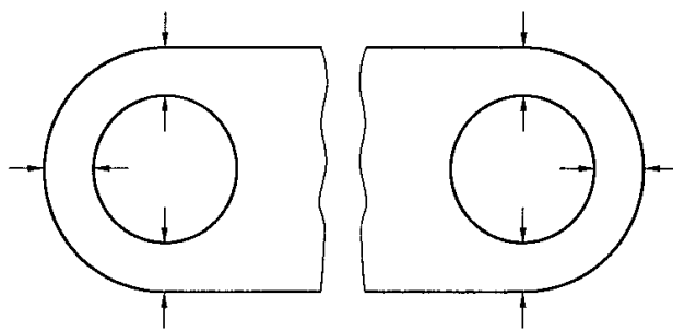
图 10 护套厚度测量(扁平带护套双芯软线)
