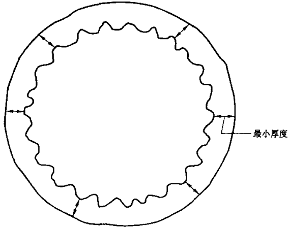
图 7 护套厚度测量(不规整圆形内表面)
