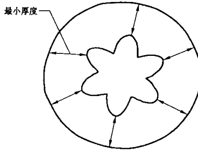
图 4 绝缘厚度测量(绞合导体)
