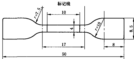
图 13 小哑铃试件
