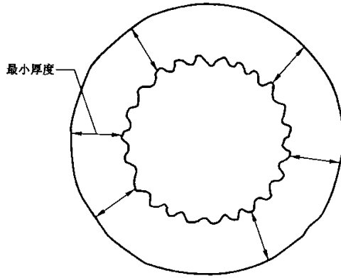
图 3 绝缘厚度测量(绞合导体)
