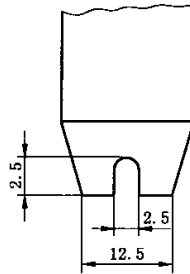
图 14 带凹槽的冲头一端
