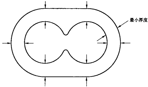
图 10 护套厚度测量(扁平带护套双芯软线)
