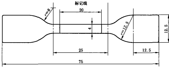
图 12 哑铃试件
