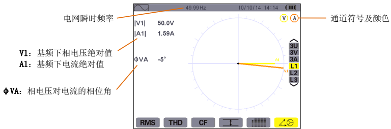
图 8-21 L1 下矢量图显示屏幕
