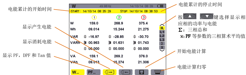
图 11-1 功率和电能屏幕
