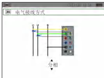
图 4-5 分相连接
