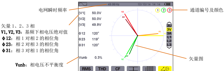
图 8-20 3V 下矢量图显示屏幕
