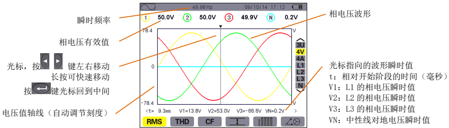
图 8-3 4V 下 RMS 显示屏幕
