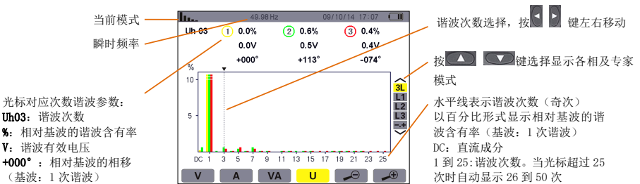
图 7-8 线电压谐波 3L 显示
