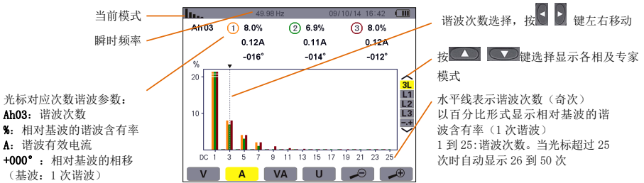
图 7-4 电流谐波 3L 显示
