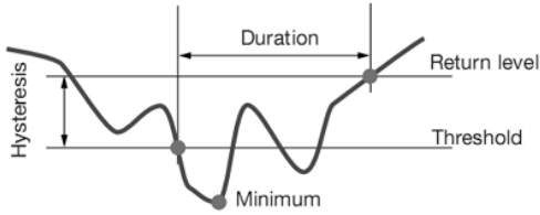
图 17-2 骤降侦测回差图例
