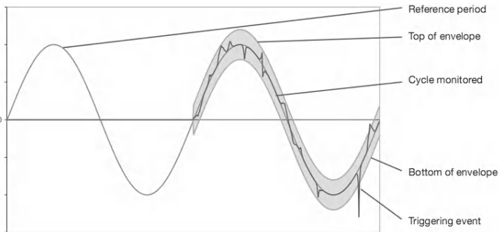
图 17-4 暂态捕捉触发原理解
