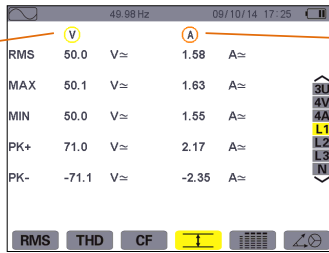
图 8-15 L1 下 Max.-Min. 显示屏幕
