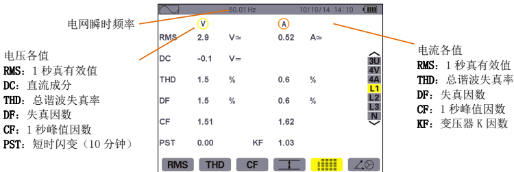
图 8-19 L1 下各值同时显示屏幕
