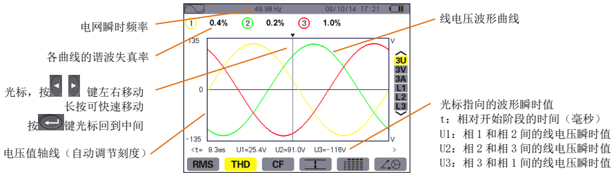
图 8-6 3U 下 THD 显示屏幕
