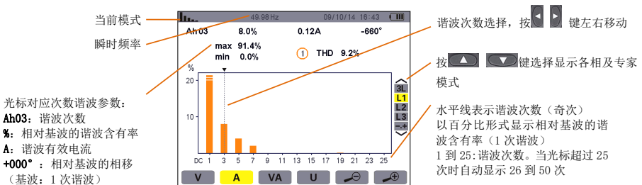
图 7-5 电流谐波 L1 显示
