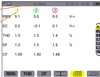
图 8-16 3U 下各值同时显示屏幕
