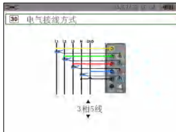
图 5-6 电气连接方式选择
