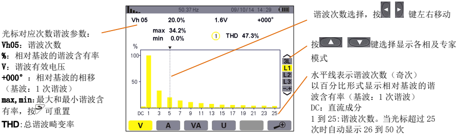
图 7-3 相电压谐波 L1 显示
