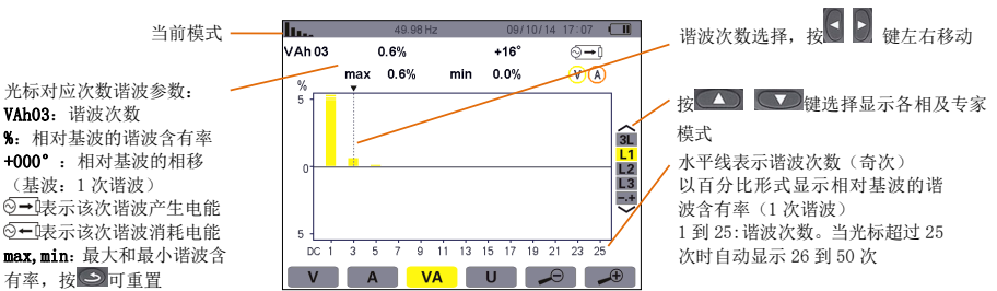
图 7-7 视在功率谐波 L1 显示
