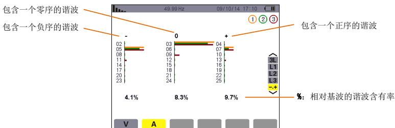
图 7-11 电流的专家模式显示
