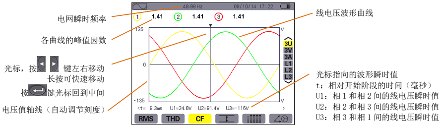
图 8-9 3U 下 CF 显示屏幕
