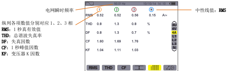
图 8-18 4A 下各值同时显示屏幕
