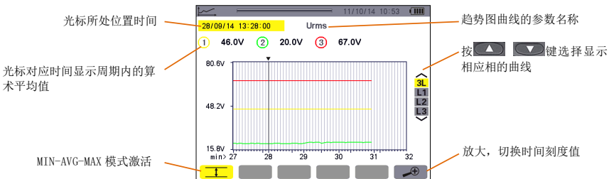
图 10-11 线电压有效值包括最大、最小、平均值
