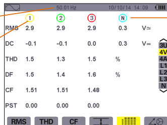
图 8-17 4V 下各值同时显示屏幕
