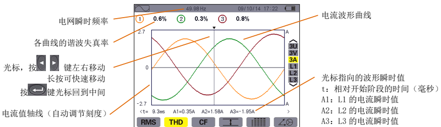
图 8-8 3A 下 THD 显示屏幕
