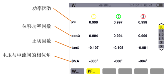
图 11-4 三相 (3L) 功率因数屏幕显示
