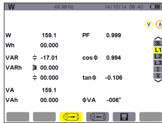
图 11-3 L1 相电能消耗显示屏幕
