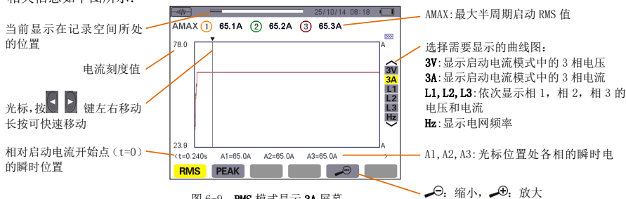
图 6-9 RMS 模式显示 3A 屏幕
