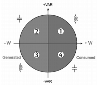
图 17-3 功率电能象限图
