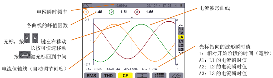
图 8-11 3A 下 CF 显示屏幕
