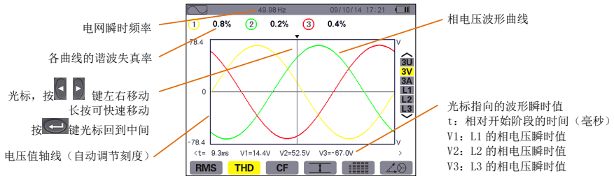
图 8-7 3V 下 THD 显示屏幕
