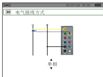
图 4-4 单相连接
