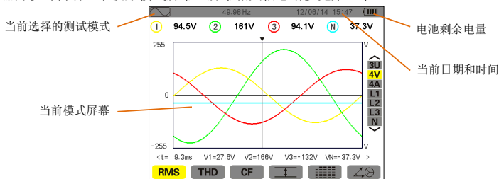
图 3-2 屏幕显示示例
