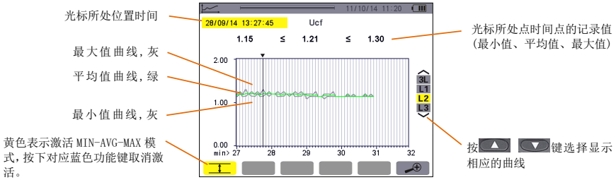
图 10-13 L2 的 Ucf 包括最大、最小、平均值
