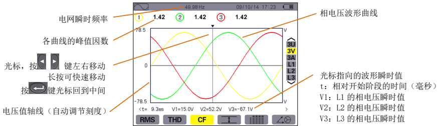
图 8-10 3V 下 CF 显示屏幕
