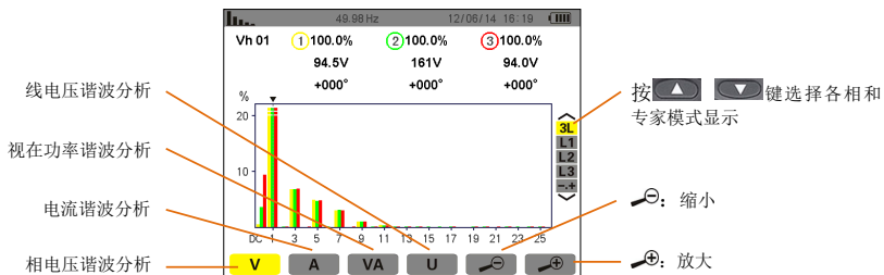
图 7-1 谐波模式屏幕
