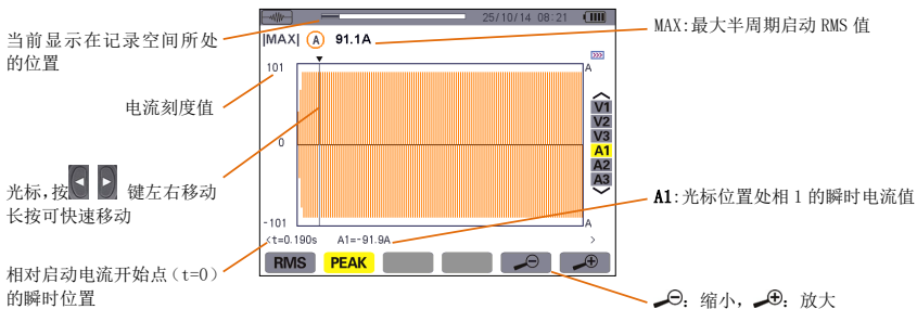
图 6-12 A1 峰值显示屏幕
