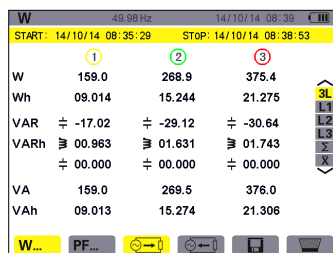
图 11-2 三相(3L)消耗电能的屏幕显示
