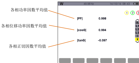
图 11-6 三相算术平均数显示屏幕
