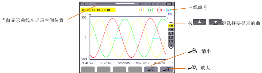
图 6-5 暂态波形曲线
