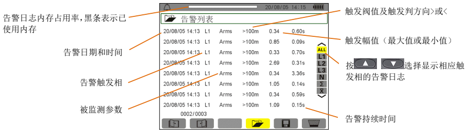
图 9-4 告警日志显示屏幕
