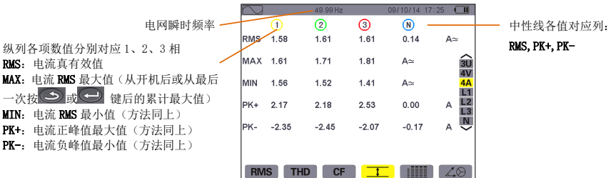
图 8-14 4A 下 Max.-Min. 显示屏幕
