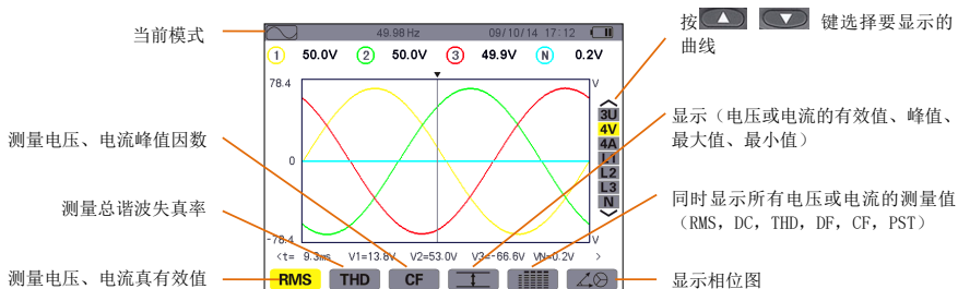
图 8-1 波形模式屏幕
