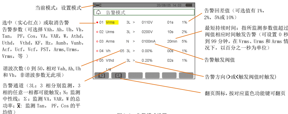
图 9-2 告警模式设置
