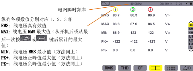
图 8-12 3U 下 Max.-Min. 显示屏幕
