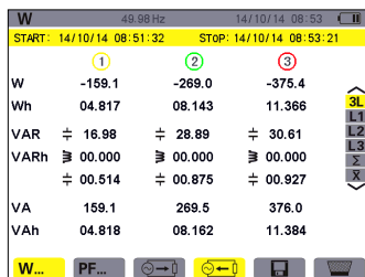
图 11-7 三相(3L)电能产生显示屏幕
