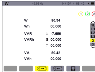
图 11-5 电能消耗三相总和显示屏幕
