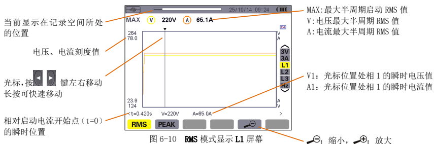
图 6-10 RMS 模式显示 L1 屏幕
