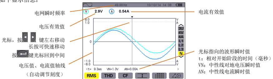
图 8-5 RMS 显示中性线屏幕
