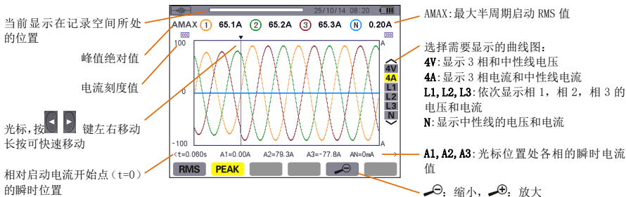
图 6-11 4A 峰值显示屏幕
