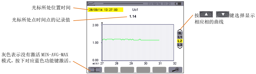
图 10-12 L2 的 Ucf 不包括最大、最小、平均值
