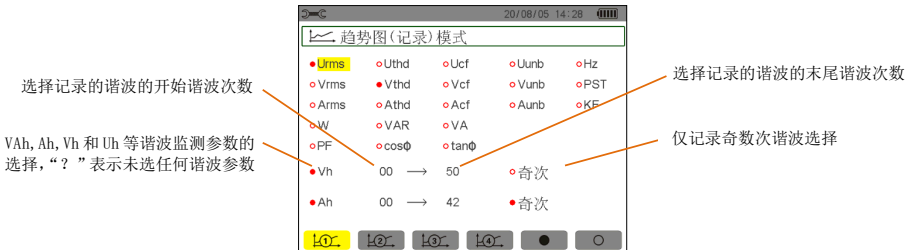
图 10-6 趋势图记录的谐波参数设定
