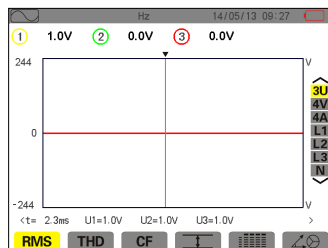
图 4-1 波形图屏幕
