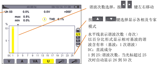
图 7-9 线电压谐波 L1 显示
