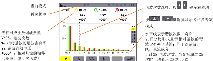
图 7-2 相电压谐波 3L 显示
