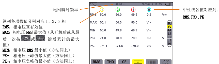
图 8-13 4V 下 Max.-Min. 显示屏幕
