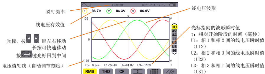
图 8-2 3U 下 RMS 显示屏幕
