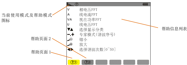
图 13-1 谐波模式下帮助页面图例，第一页
