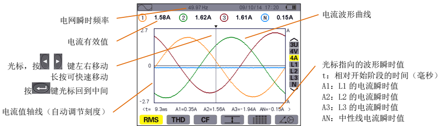
图 8-4 4A 下 RMS 显示屏幕
