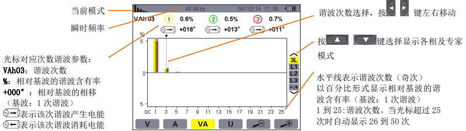
图 7-6 视在功率谐波 3L 显示
