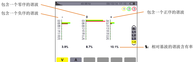
图 7-10 相电压的专家模式显示
