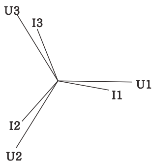
三相四线向量图
