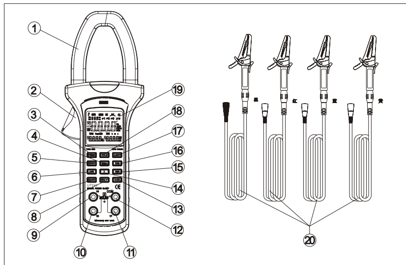
图1 仪表正视图
