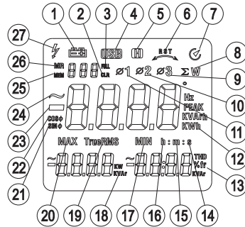
图3 LCD全显图
