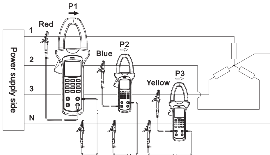
图4 三相四线制功率测量 P=P_1+P_2+P_3
