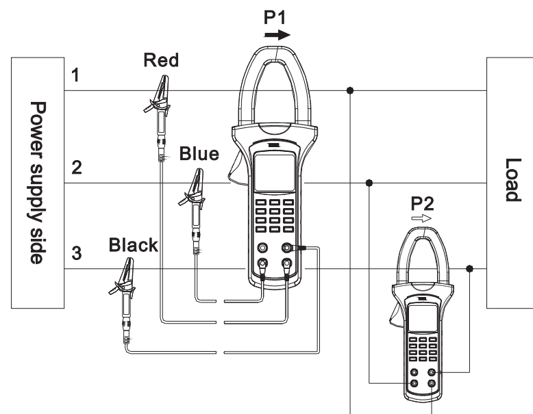
图5 三相三线制功率测量 P=P_1+P_2
