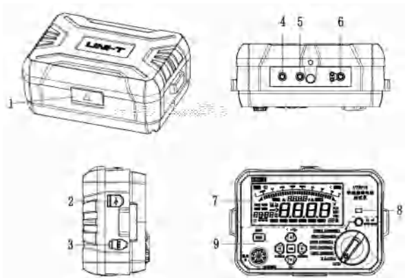
图7.1 仪表外观示意图
