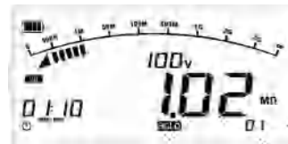
图13.4 100V档停止连续测试界面
