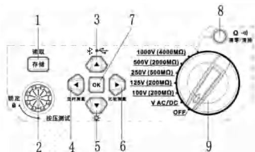
图8. 1功能按键及刀盘布局示意图
