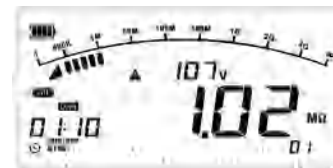
图13.3 100V档开启连续测试界面
