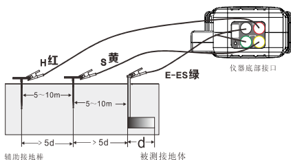
图 8.4-2 三线法测量接线示意图
