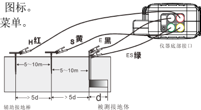
图 8.4-1 四线法测试接线示意图
