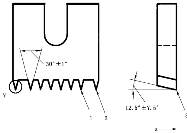
b) 使用电动驱动装置的多刃切割刀具
