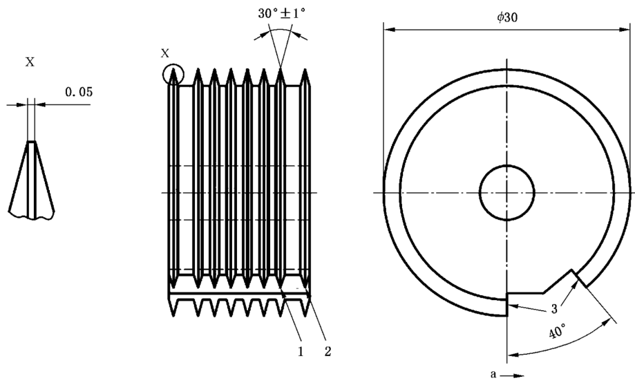
a) 手动多刃切割刀具
