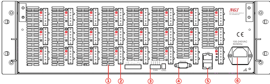
图 3-19 后面板
