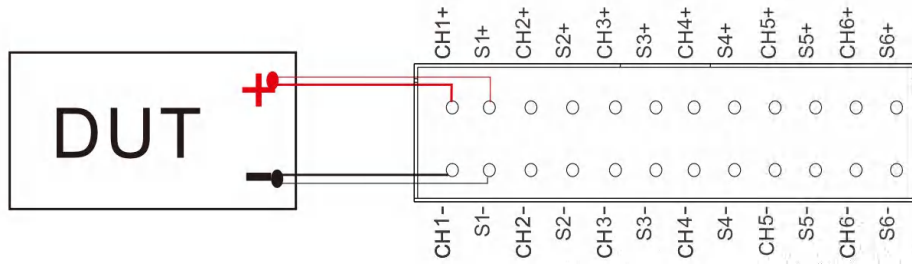
图 3-28 接线图
