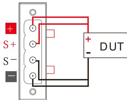
图 3-27 接线图
