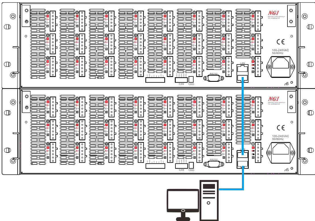
图 3-24 多机控制接线图
