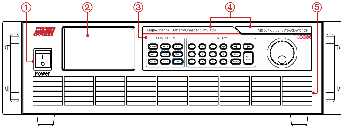
图 3-14 前面板
