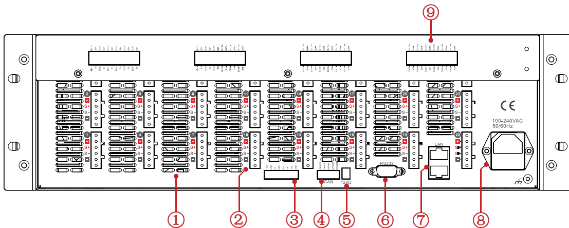
图 3-20 后面板
