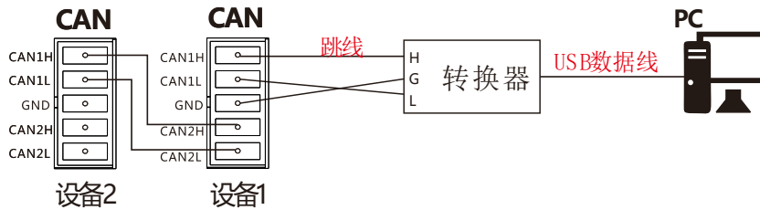
图 3-26 连接示意图
