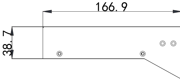
图 3-8 侧视尺寸
