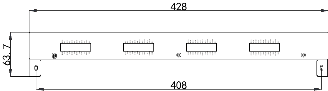
图 3-9 后面板尺寸
