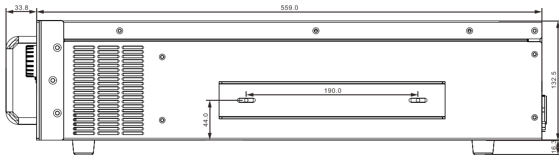
图 3-2 机箱侧视尺寸
