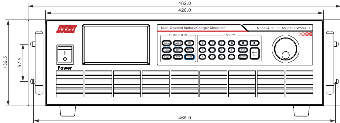
图 3-4 前面板尺寸
