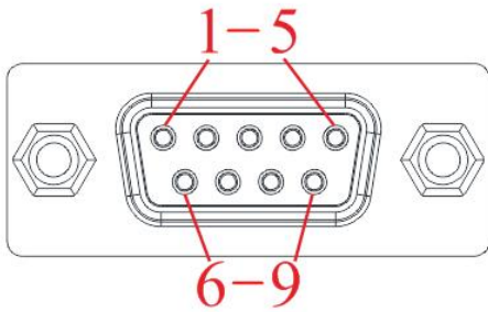
图 3-23 RS232 引脚标识
