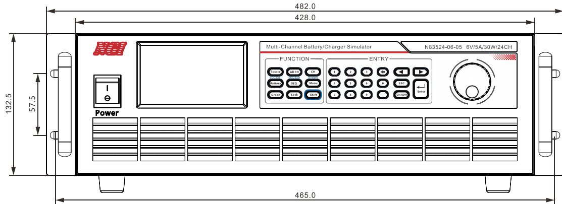
图 3-1 前面板尺寸
