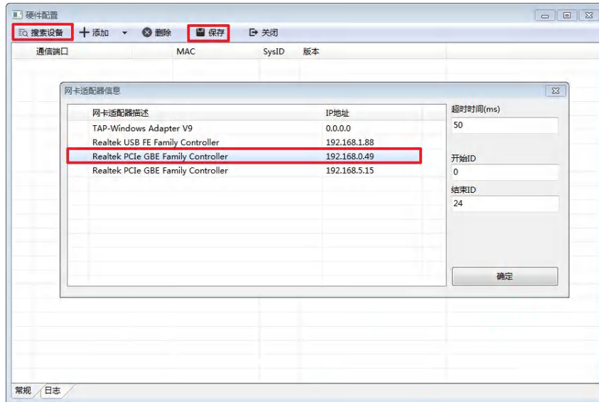
图 4-24 搜索设备
