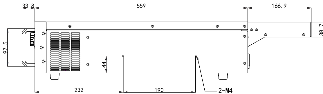
图 3-5 机箱侧视尺寸
