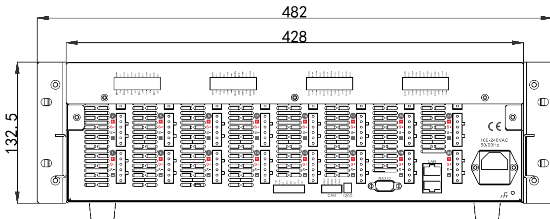
图 3-6 后面板尺寸
