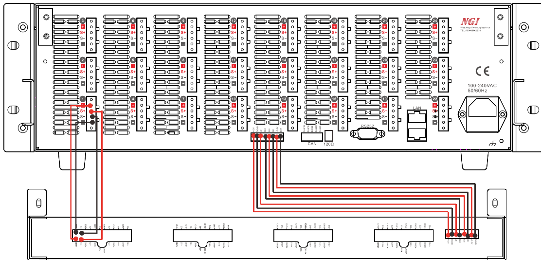
图 3-11 线束连接
