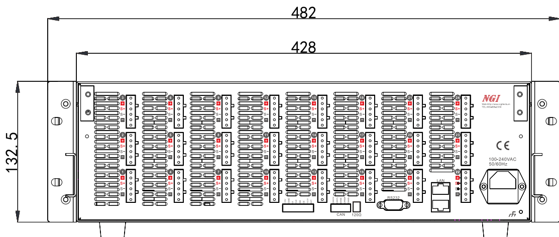
图 3-3 后面板尺寸
