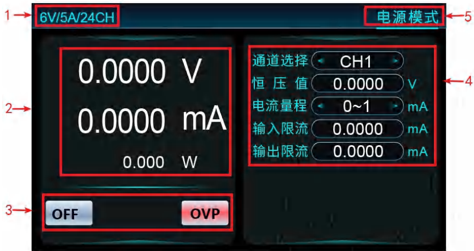
图 5-2 界面介绍
