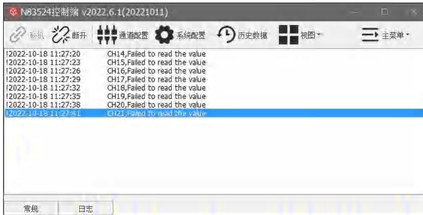
图 4-22 日志
