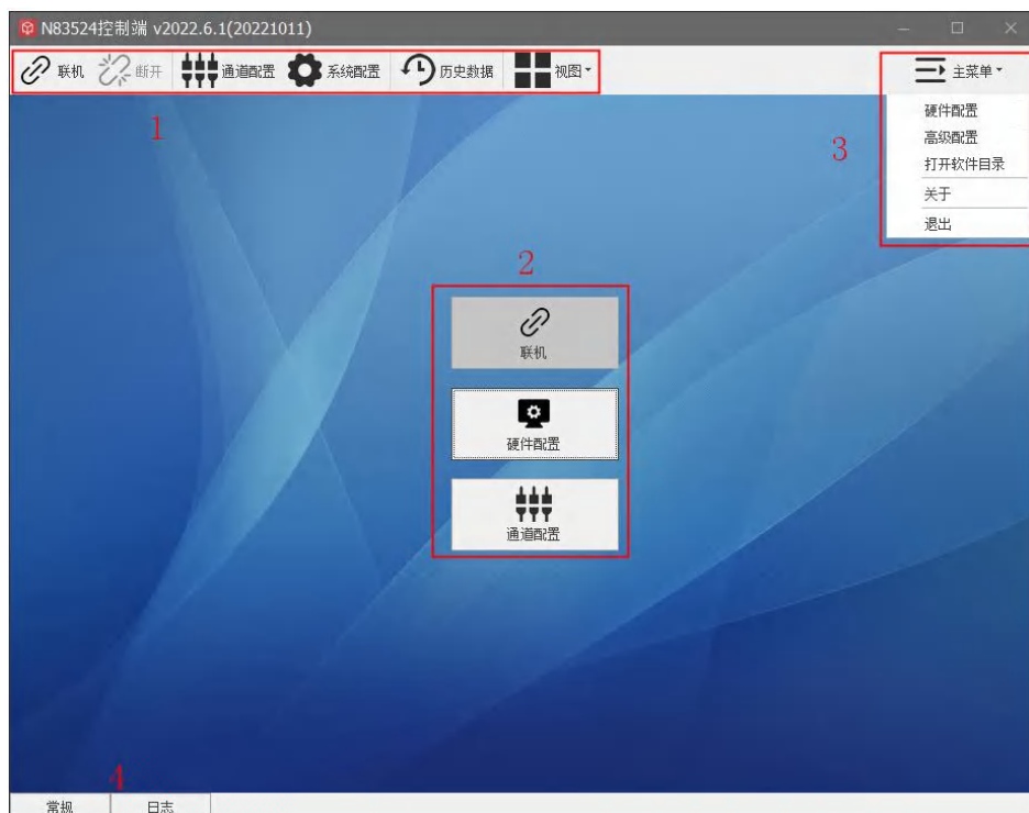
图 4-21 程序主界面
