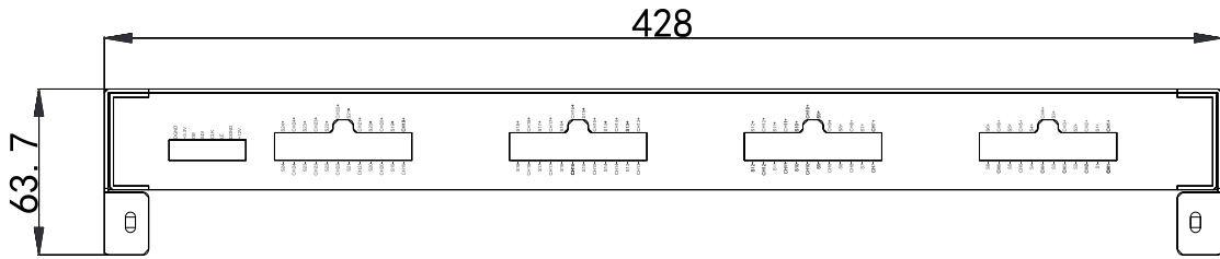
图 3-7 与 N83624 连接端尺寸
