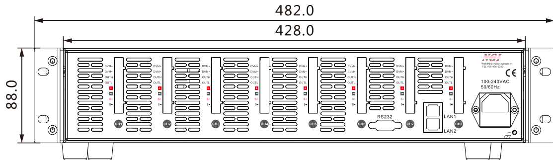
图 3-3 后面板尺寸
