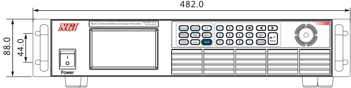
图 3-1 前面板尺寸
