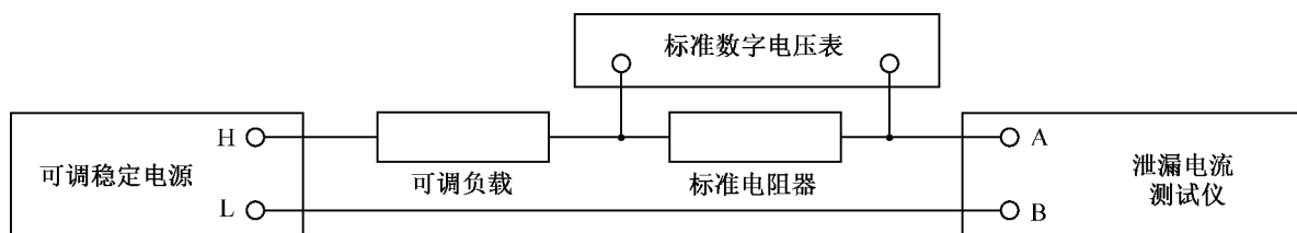
图 2 标准数字电压表法
