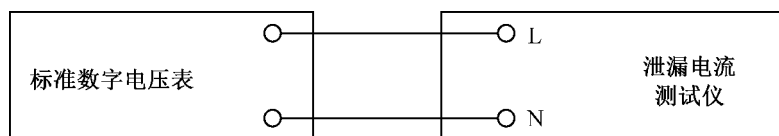
图 6 自身提供试验电压的测试仪的试验电压检定线路图
