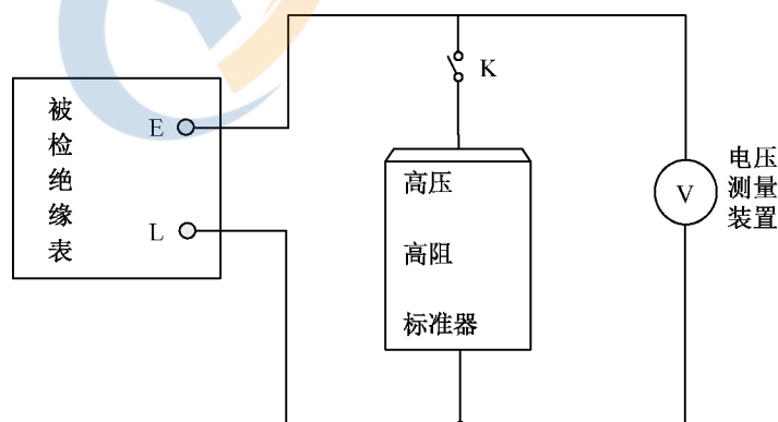
图4 测量端子电压检定接线图
