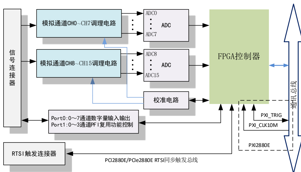
图2-2-1 2880E 系统框图
