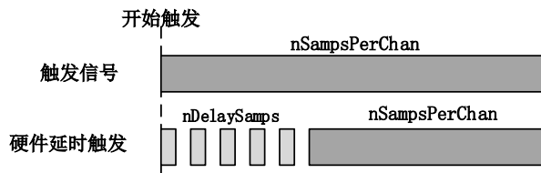
图 7-2-3 AI 硬件延时触发
