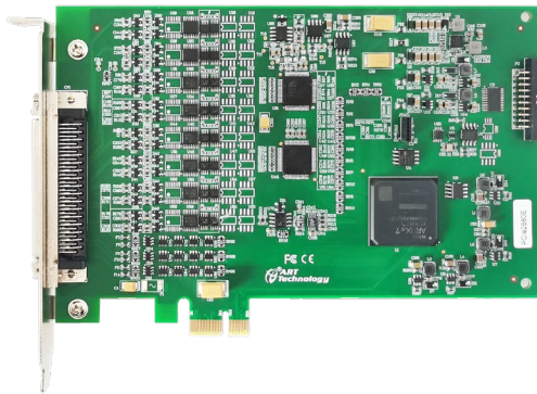
图 3-1-2 PCIe2880E 板卡外形图
