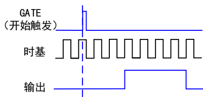
图 5-8-2 具有启动触发的单脉冲生成
