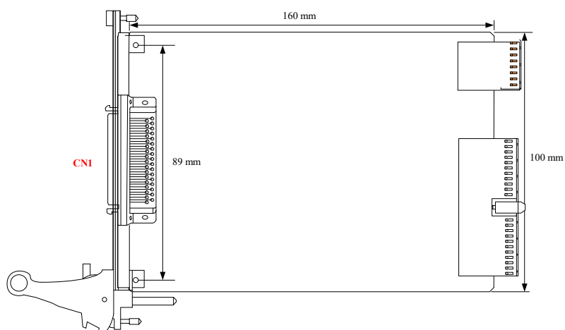
图 3-2-3 PCI2880E 板卡尺寸图
