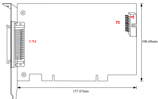
图 3-2-1 PCI2880E 板卡尺寸图
