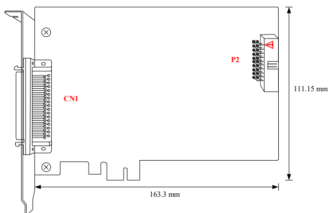
图 3-2-2 PCI2880E 板卡尺寸图
