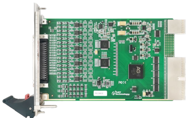
图 3-1-3 PXI2880E 板卡外形图
