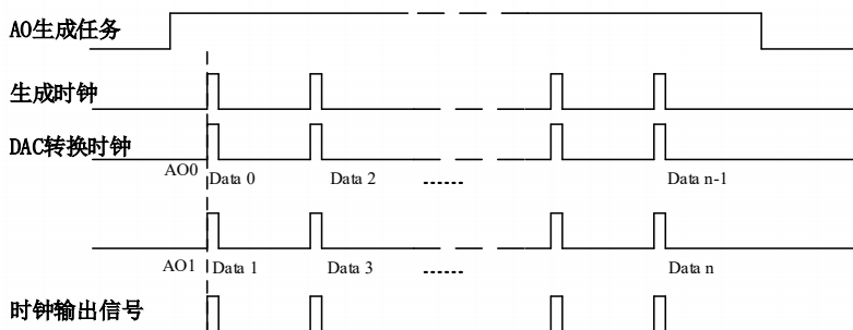
图 5-6-2 内时钟时序图
