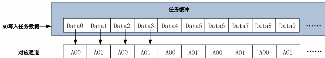
图 5-5-2 AO 多通道存储顺序
