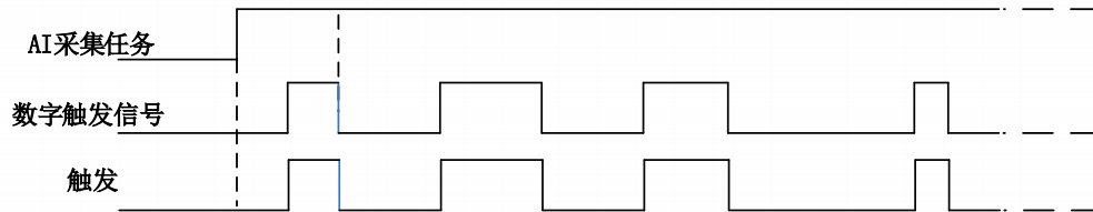
图8-3-9 数字边沿触发--下降沿触发
