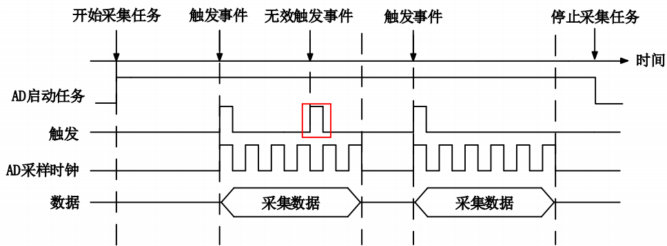
图 8-2-5 上升沿重触发
