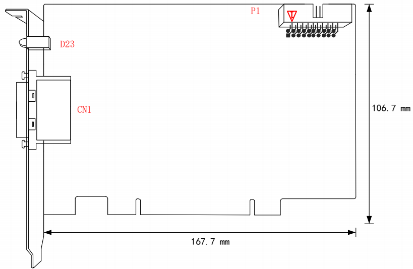
图 3-2-1 PCI 977X 板卡尺寸图
