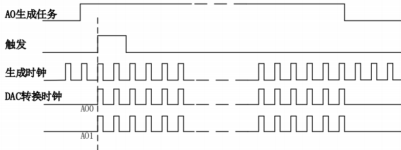
图 5-7-3 内、外时钟连续生成
