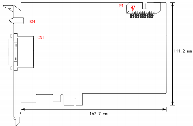
图 3-2-2 PCIe 977X 板卡尺寸图
