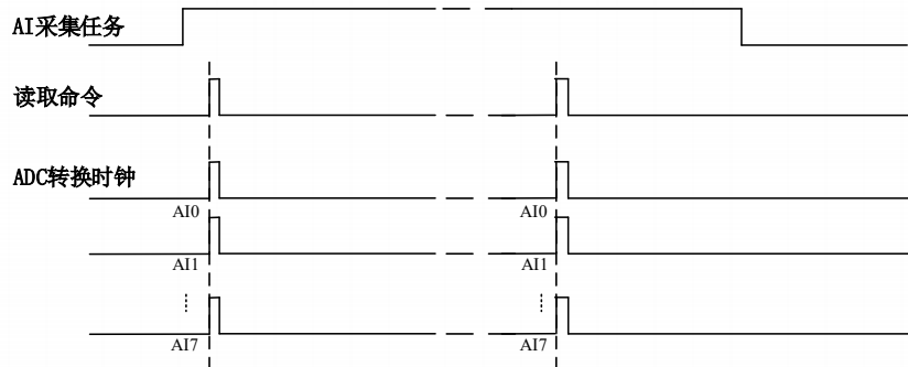
图4-7-1 按需单点采集
