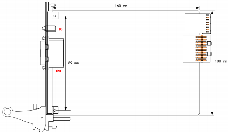
图 3-2-4 PXIe 977X 板卡尺寸图
