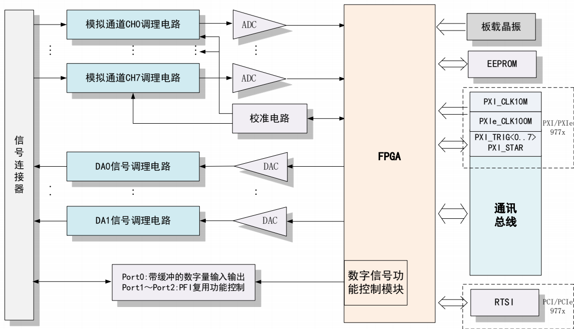
图2-2-1 977X系统框图
