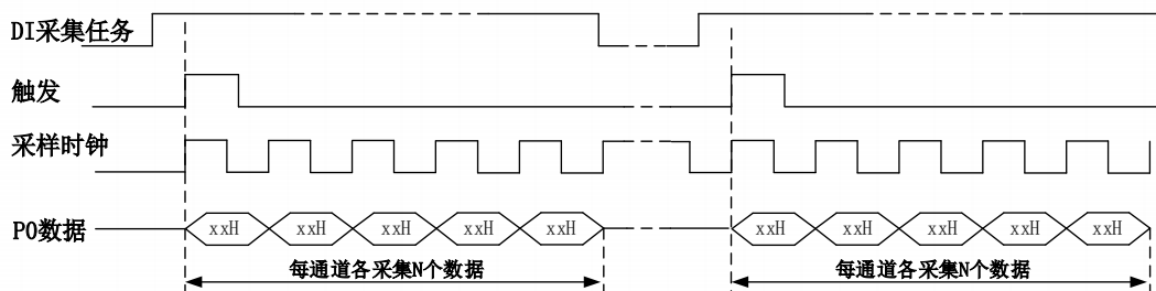
图 7-5-2 有限点采样
