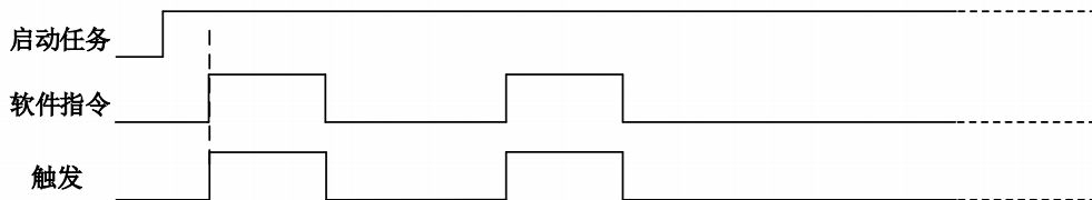
图8-3-2 AI软件强制触发
