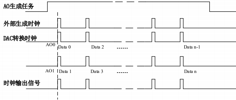
图 5-6-3 外时钟时序图
