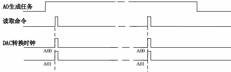
图 5-7-1 按需单点采集
