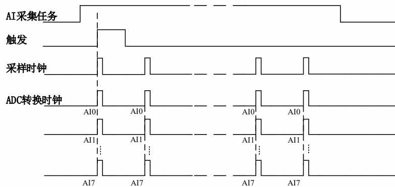
图4-7-3 时钟连续采样
