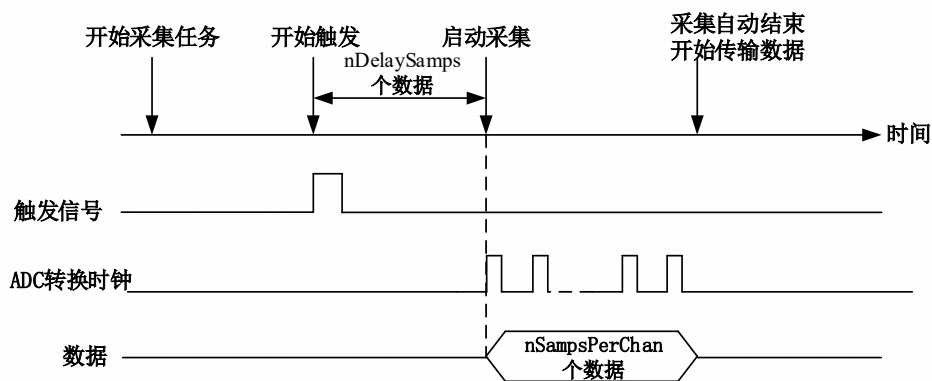
图 8-2-3 硬件延时触发
