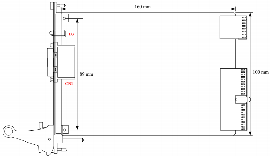
图 3-2-3 PXI 977X 板卡尺寸图
