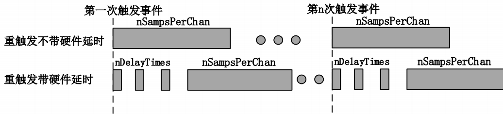
图 8-2-4 重触发
