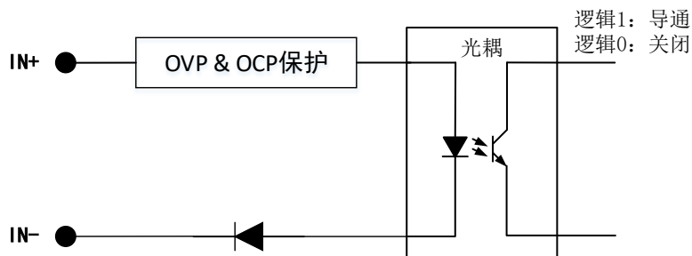
图3-4-1 输入端电路
