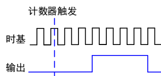
图 4-8-1 单脉冲生成
