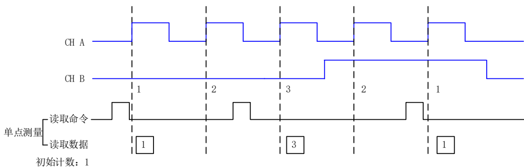
图 4-7-5 单脉冲编码
