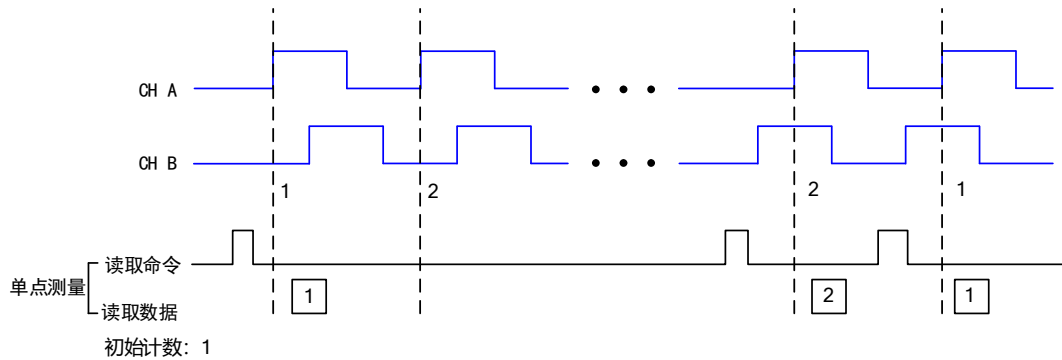
图 4-7-1 X1 编码
