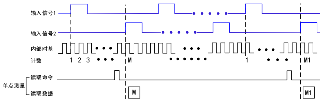
图 4-6-1 两边沿均上升沿有效示意图
