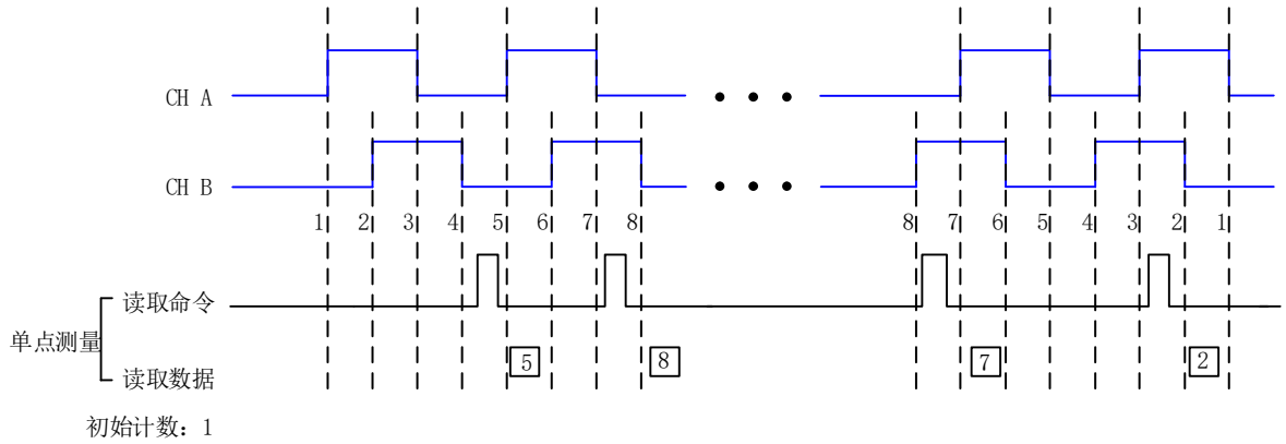
图 4-7-3 X4 编码
