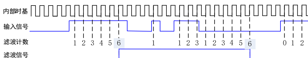
图 4-9-1 数字滤波
