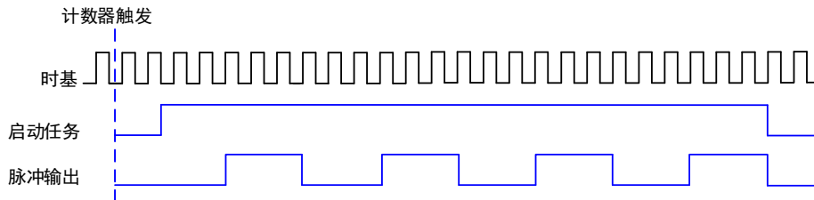
图 4-8-3 有限脉冲序列生成
