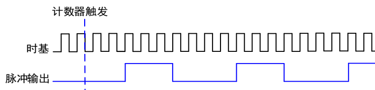
图 4-8-6 连续脉冲序列生成
