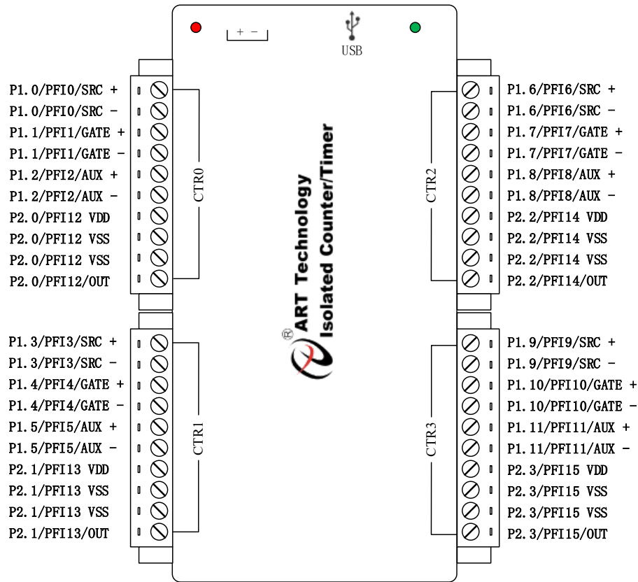
图3-3-1 管脚定义
