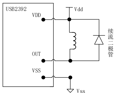
图 3-5-6 外接感性负载连接示意图
