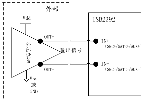
图3-5-2 差分输入信号接线方法
