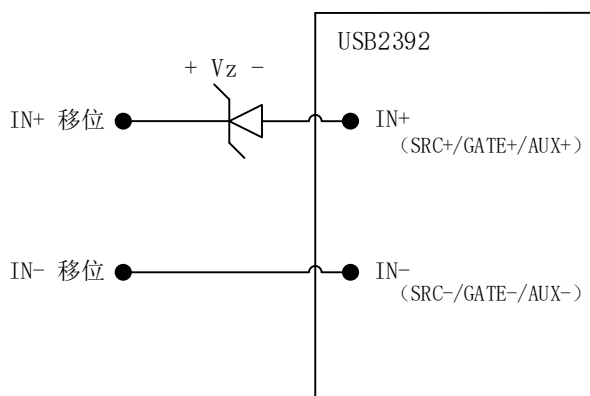
图 3-6-1 外接稳压二极管连接示意图
