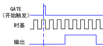
图 4-8-2 具有开始触发的单脉冲生成
