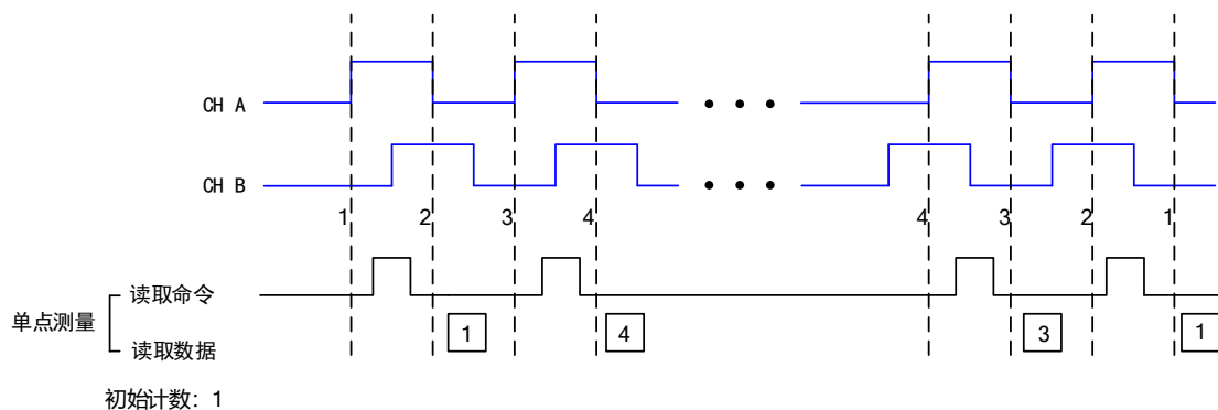
图 4-7-2 X2 编码
