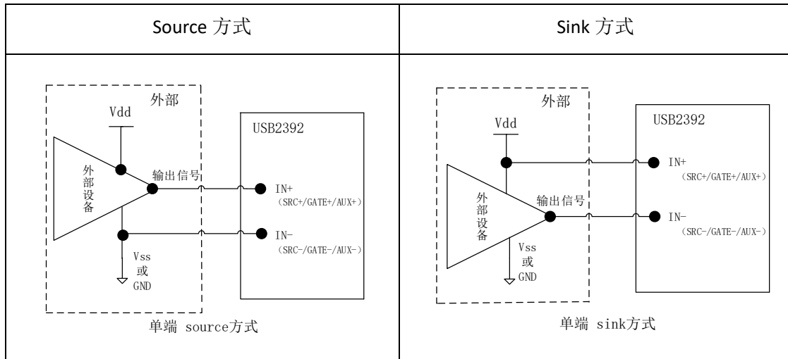
图3-5-1 单端输入信号接线方法
