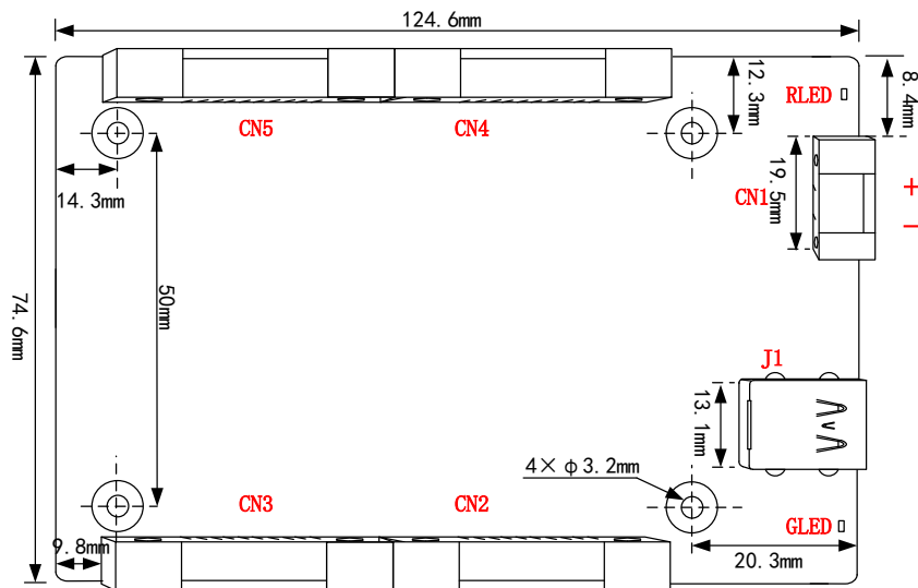
图 3-2-1 板卡尺寸图
