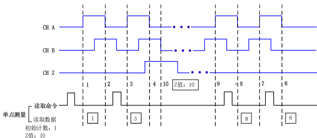
图 4-7-6 Z 索引
