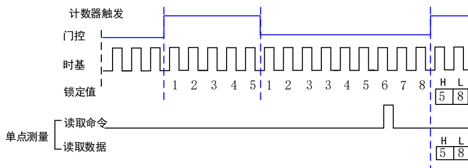
图 4-4-1 单（按需）脉冲测量
