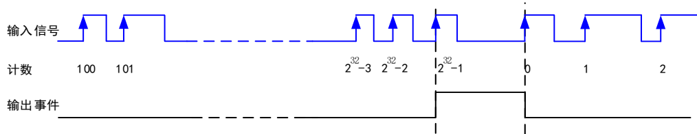
图 4-10-1 脉冲方式输出
