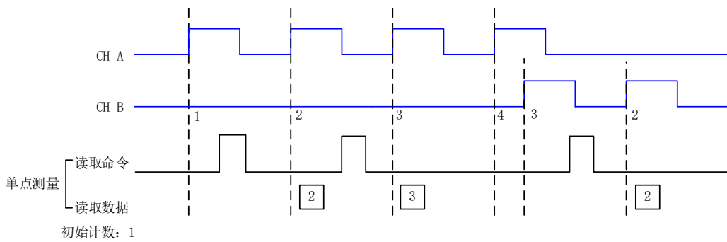
图 4-7-4 双脉冲编码
