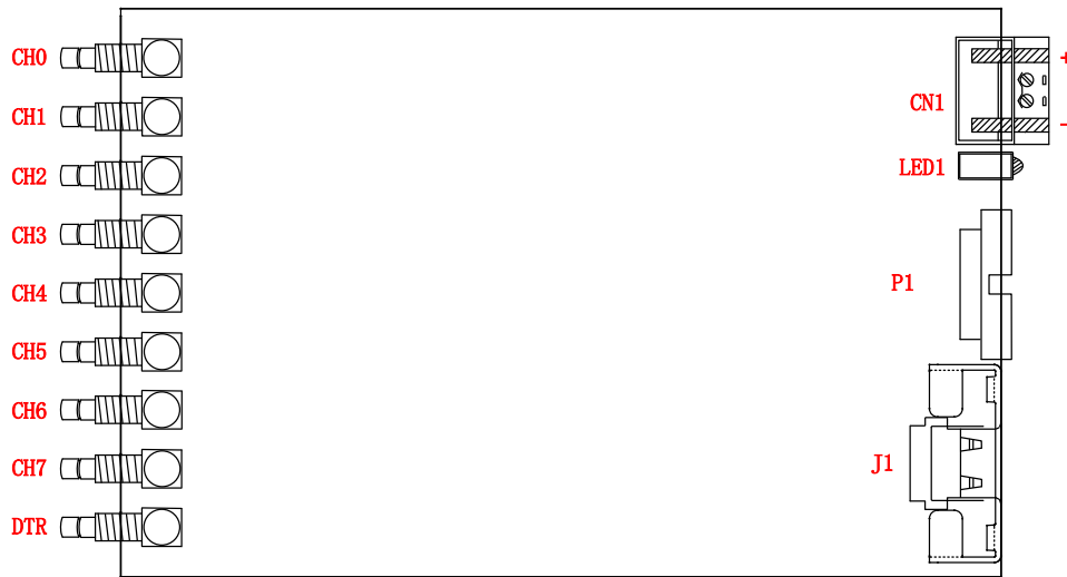
图 3-2-2 接口定义
