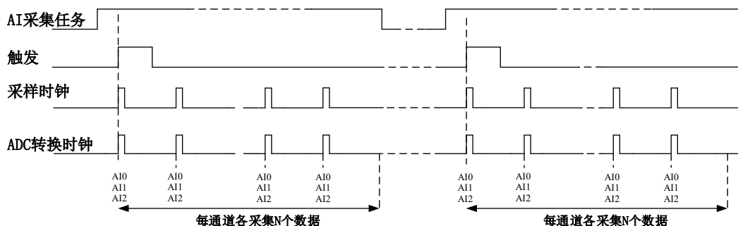
图4-6-2 有限点采样
