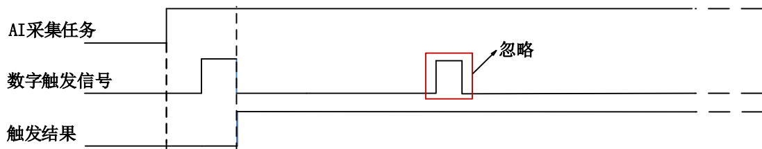
图4-8-10 数字边沿触发--下降沿触发
