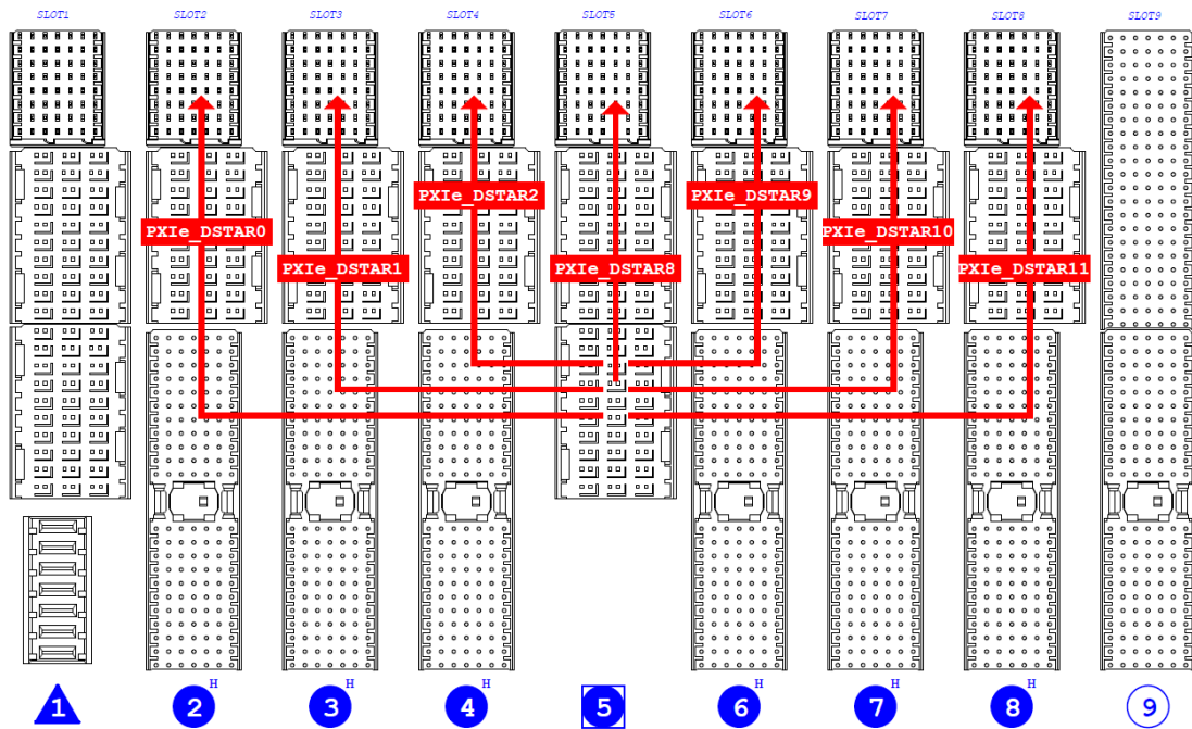
图 2-11 差分星形触发
