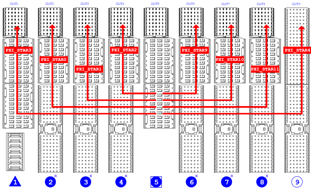
图 2-10 单端星形触发
