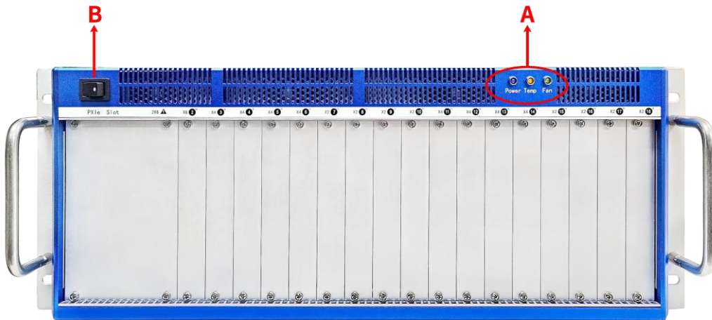
图 1 前面板图
