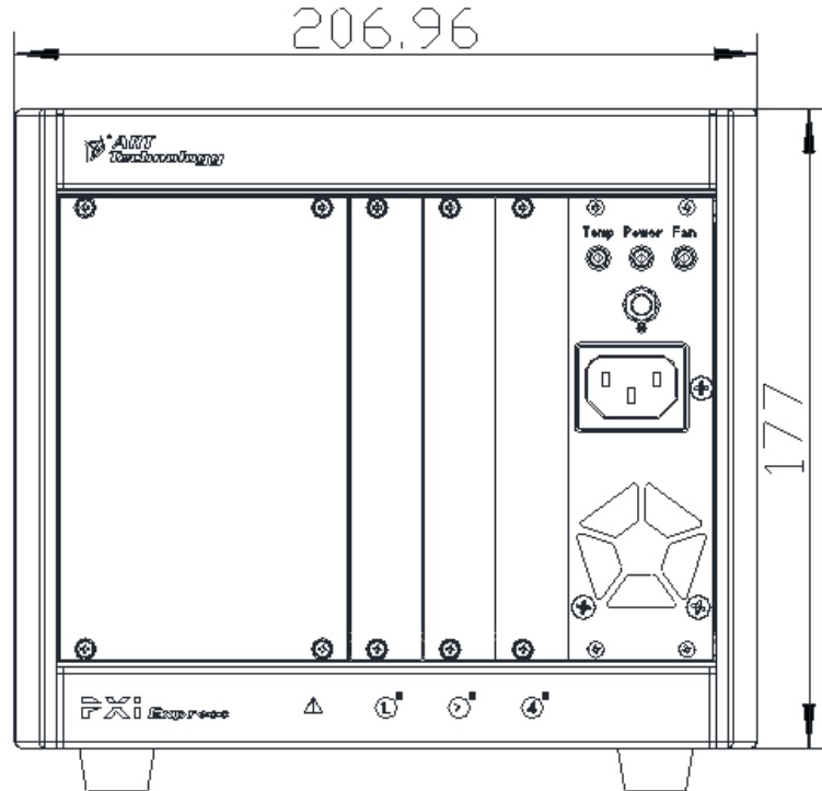
图 1 产品正视图
