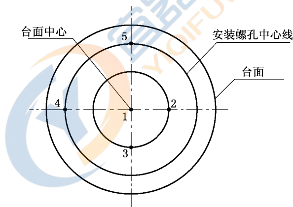
图 5 校准附加台面加速度均匀度的布点图
