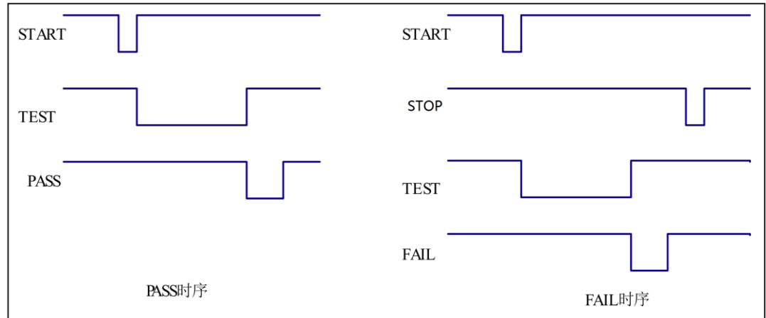
图 8-3 PLC 时序图
