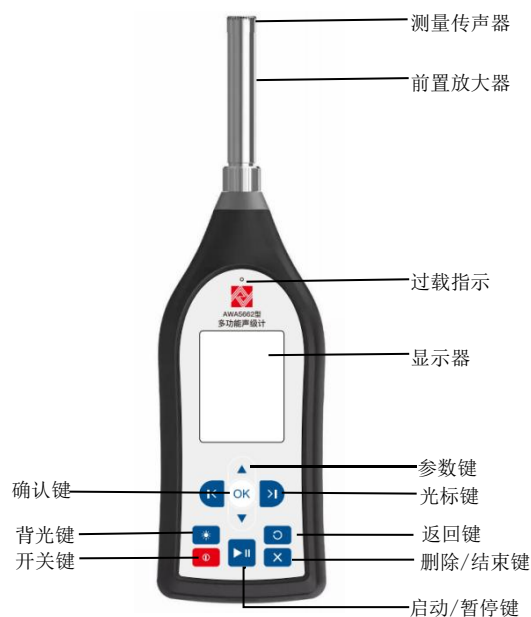
图 4-1 仪器正面
