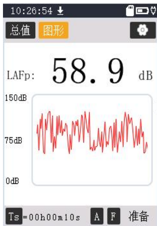
图 6-2-1-3 图形界面
