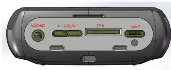
图 4-4 底部接口
