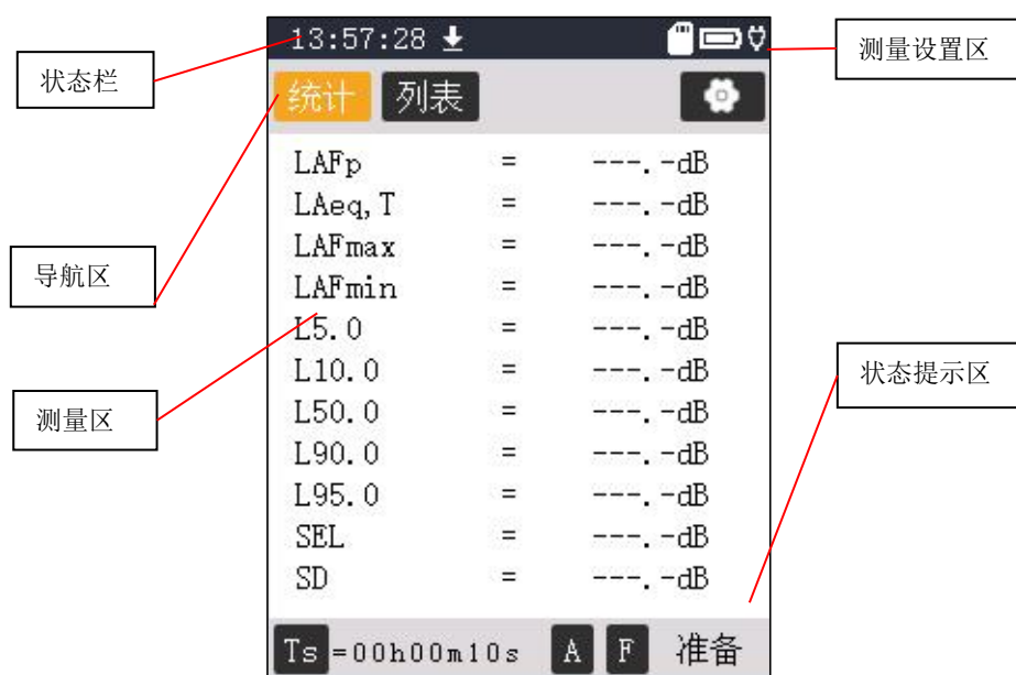
图 6-2-2-1 统计列表界面
