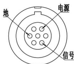
图 4-3 插座引脚
