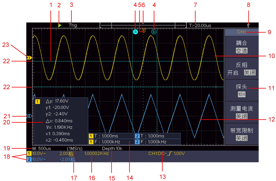
图 3-4：显示界面说明图
