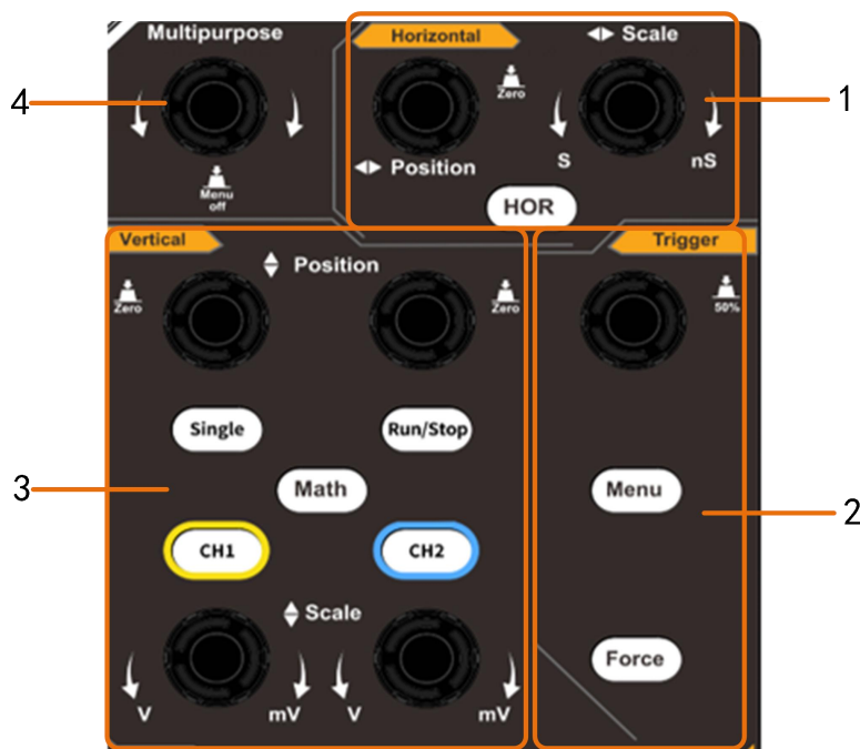
图 3-3: 按键和旋钮控制区说明图
