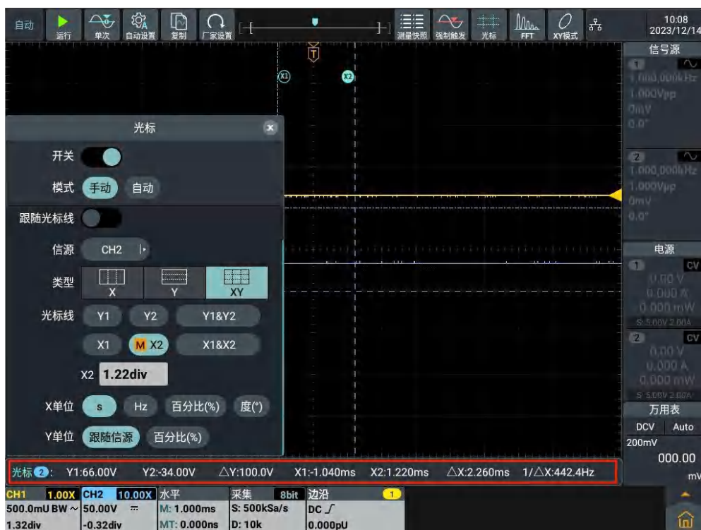
图 5-8：时间&amp;电压光标测量波形
