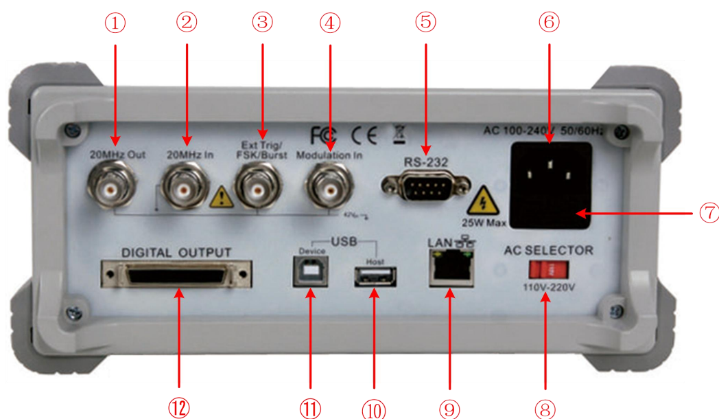
图 4-2 后面板概览
