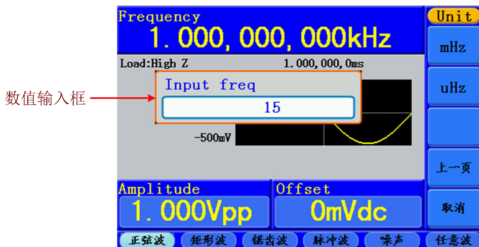
图 5-2: 使用数字键盘设置频率
