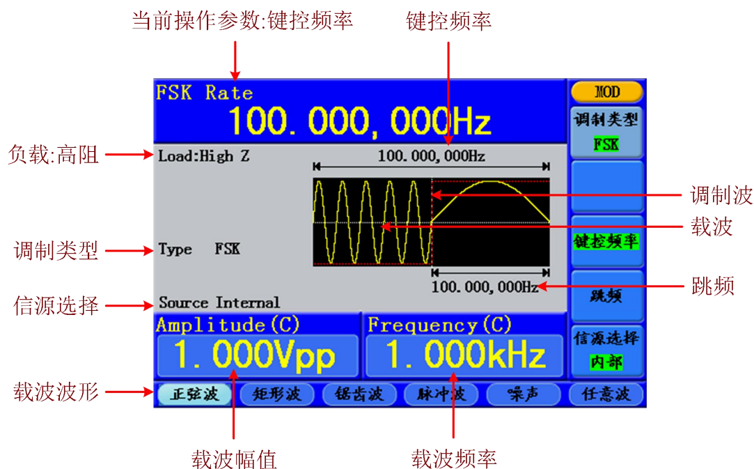
图 5-15: 频移键控调制的用户界面
