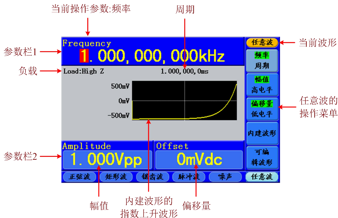
图 5-11：任意波用户界面
