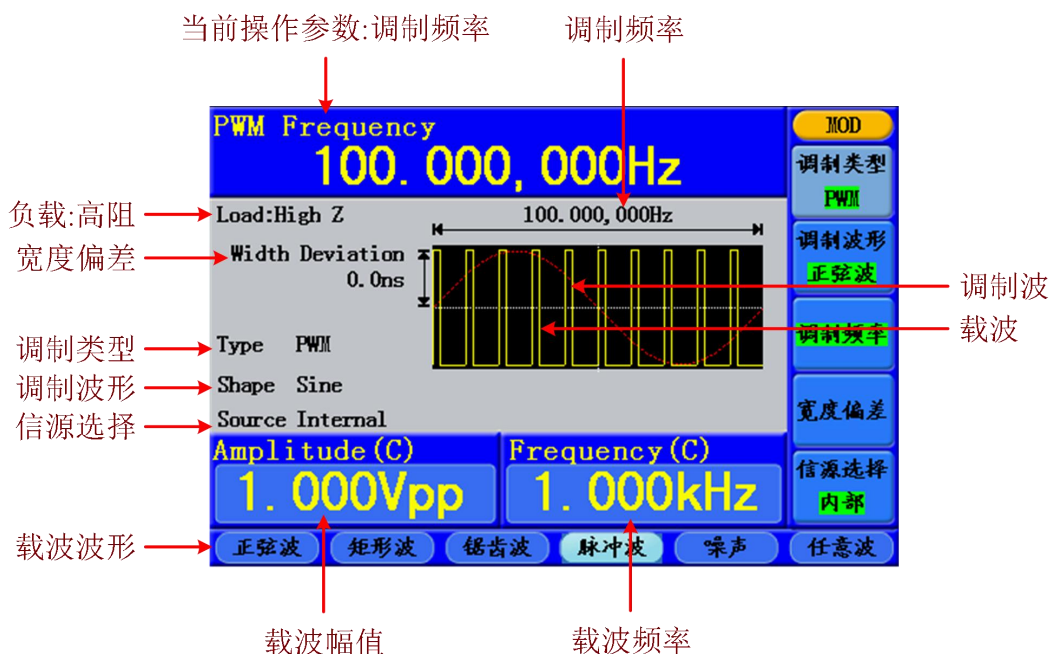
图 5-16: 脉宽调制的用户界面
