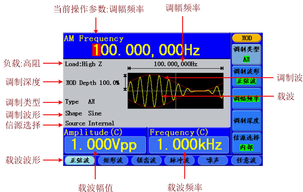
图 5-12: 振幅调制的用户界面
