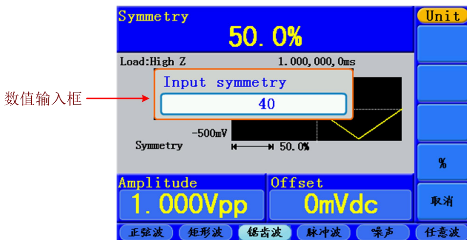
图 5-6：设置锯齿波的对称性
