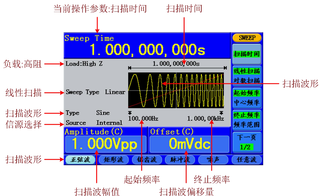
图 5-17: 扫描模式的用户界面
