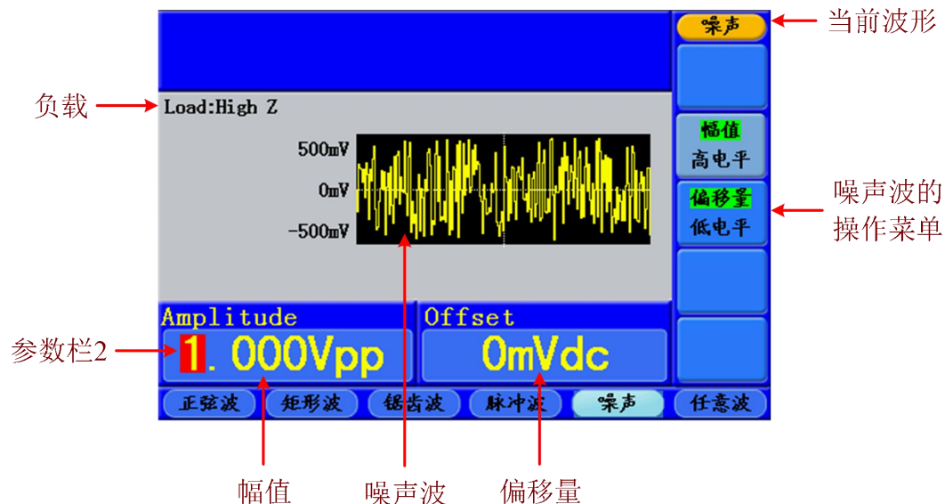
图 5-10：噪声波用户界面
