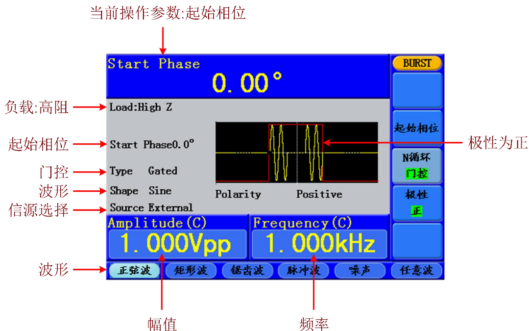
图 5-19: 门控脉冲串的用户界面
