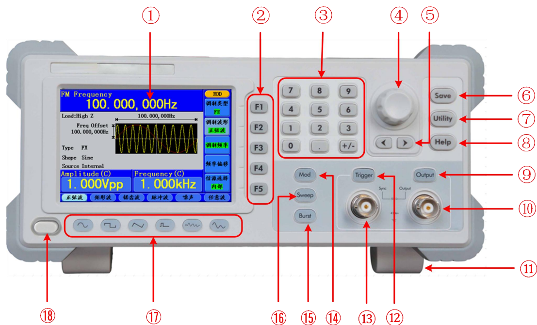
图 4-1 前面板概览
