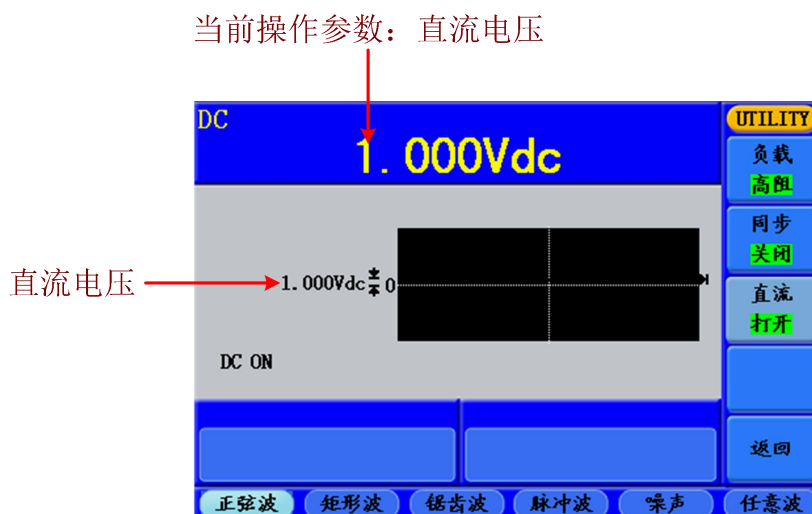
图 5-21：输出直流
