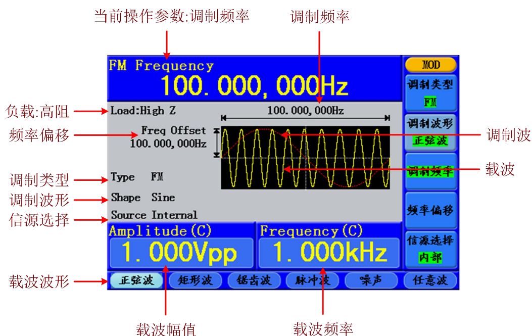
图 5-13: 频率调制的用户界面
