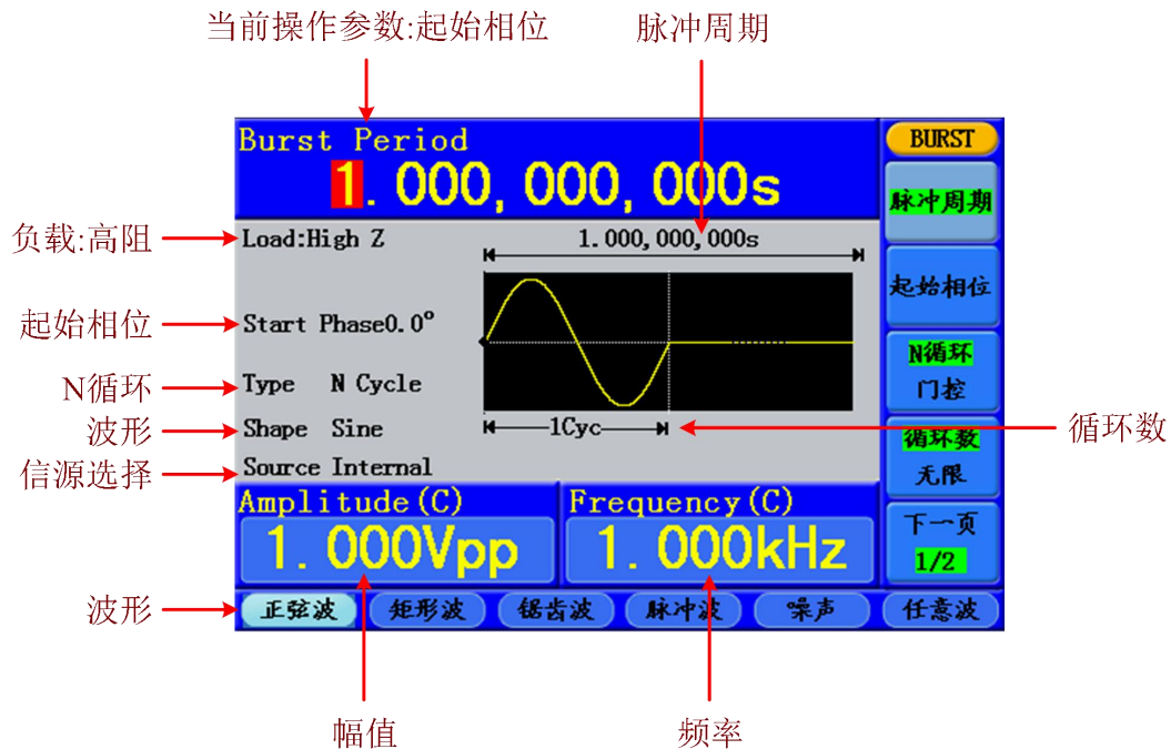
图 5-18: N 循环脉冲串的用户界面
