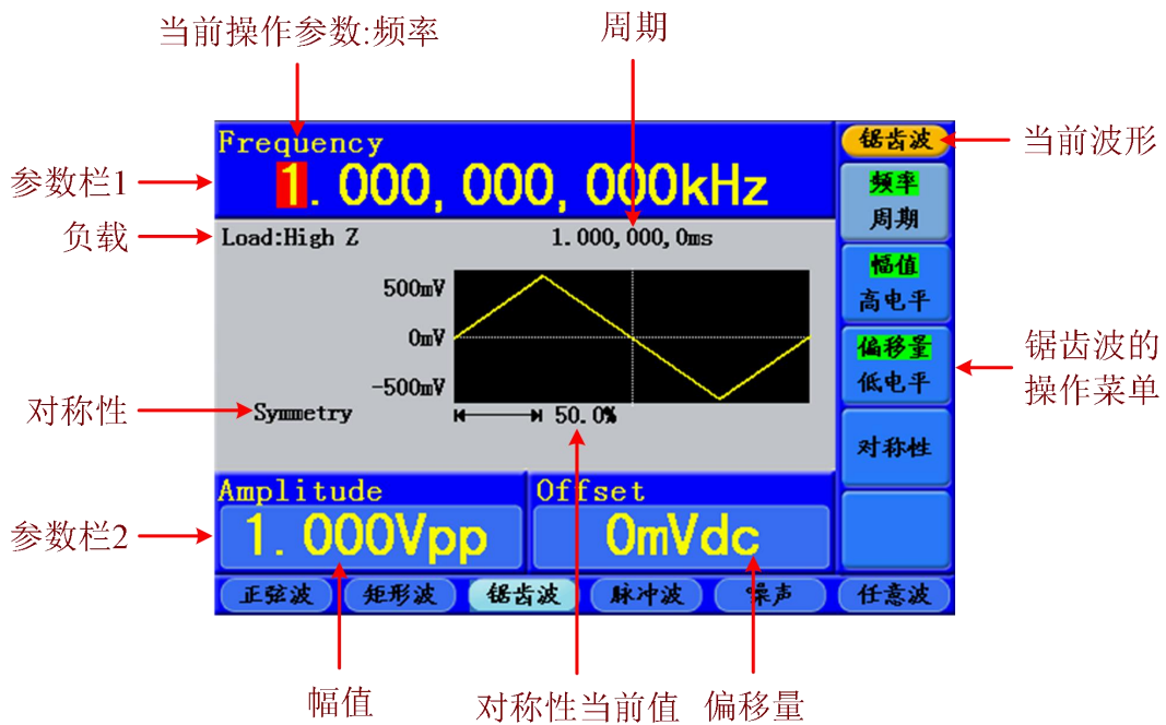
图 5-5: 锯齿波用户界面
