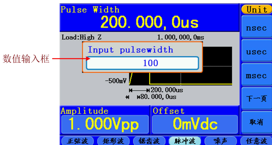
图 5-8: 设置脉冲波的脉宽
