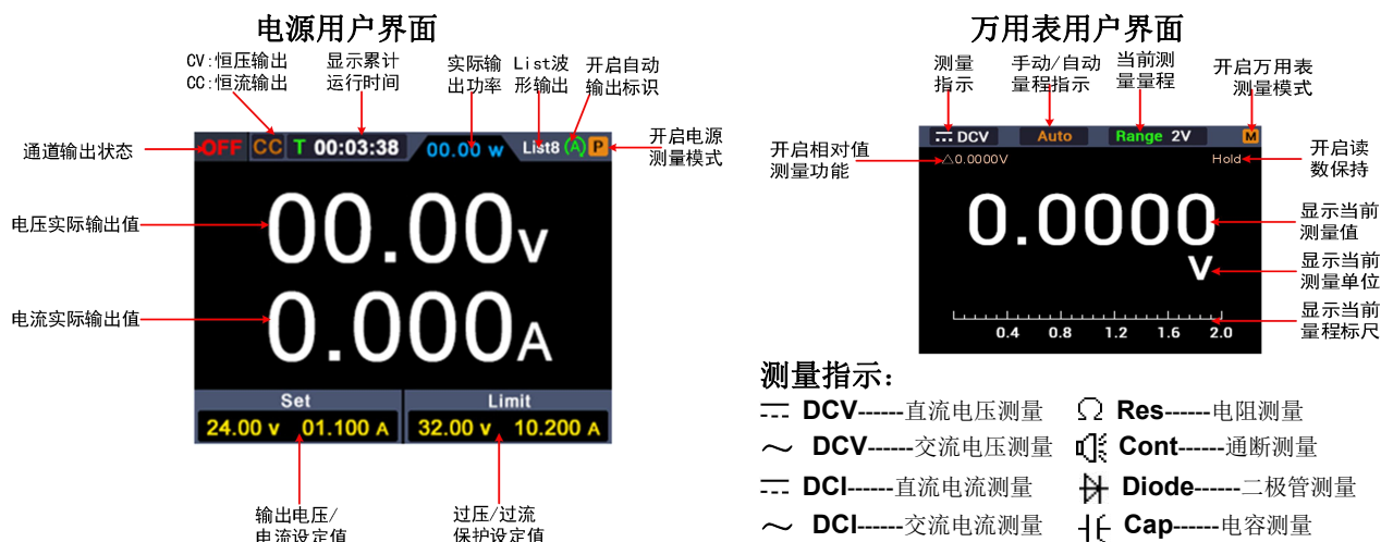
图 2-3 用户界面
