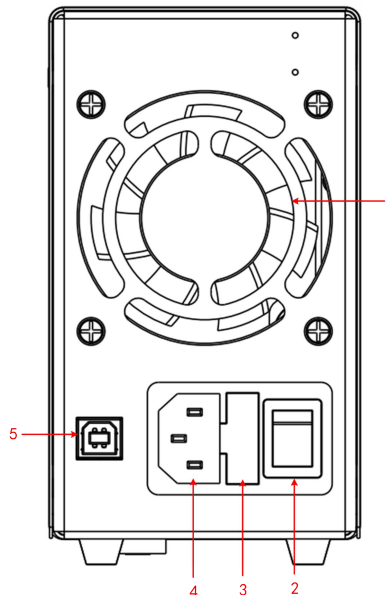
图 2-2 后面板概览
