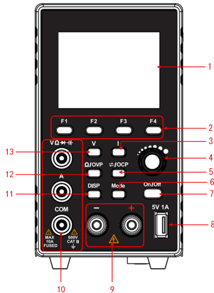
图 2-1 前面板概览
