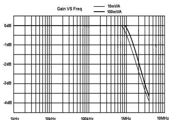
图 2 CPL8100B 典型增益频率关系曲线
