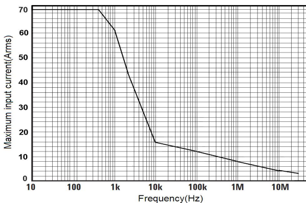
图 8 HCPX8070 最大测量电流 VS 频率曲线 (超过该曲线所示最大电流连续使用会导致探头烧毁)
