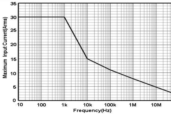
图 2.a HCPX8030 最大测量电流 VS 频率曲线
