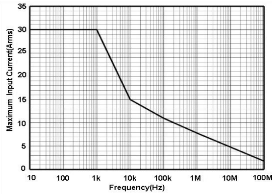
图 2.c HCPX8030D 最大测量电流 VS 频率曲线
