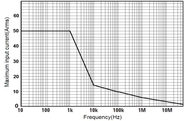
图 5 HCPX8050 最大测量电流 VS 频率曲线 (超过该曲线所示最大电流连续使用会导致探头烧毁)
