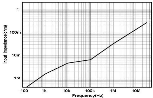
图 9 HCPX8070 输入阻抗 VS 频率曲线
