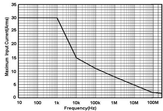
图 2.d HCPX8030H 最大测量电流 VS 频率曲线
