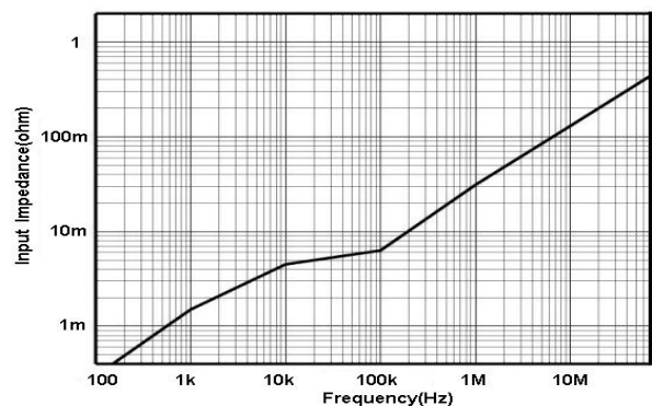
图 3.b HCPX8030C 输入阻抗 VS 频率曲线
