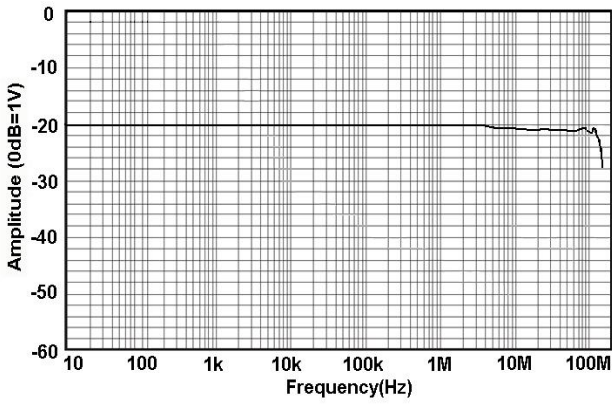
图 1.c HCPX8030D 幅频曲线
