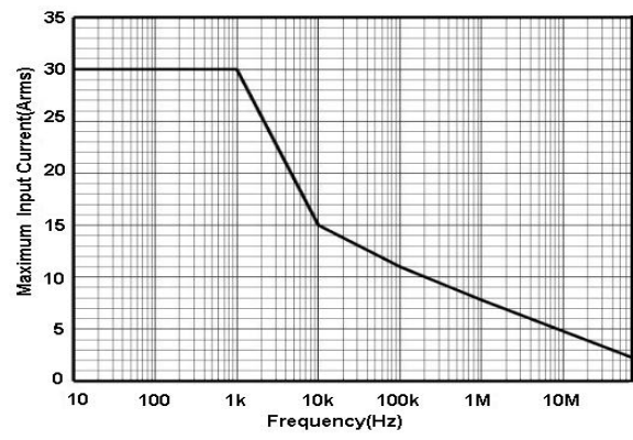
图 2.b HCPX8030C 最大测量电流 VS 频率曲线
