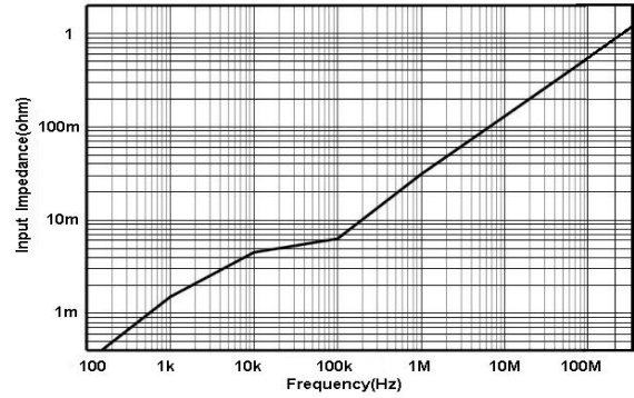
图 3.d HCPX8030H 输入阻抗 VS 频率曲线
