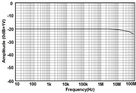
图 4 HCPX8050 幅频曲线
