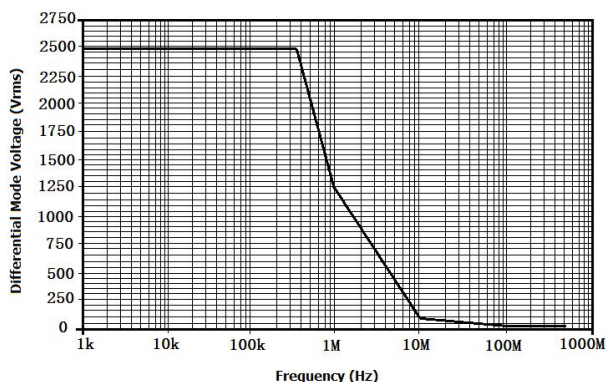
图 3 DPR6350A 最大差模电压 VS 频率
