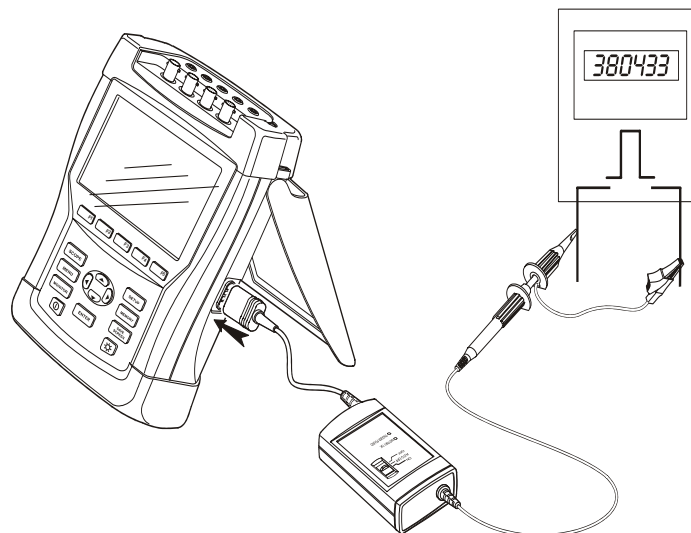
图 11-1. 利用脉冲输出验证能量计
