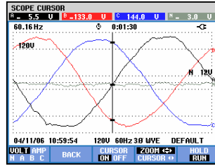
图 19-3. 波形显示（光标和缩放功能启用）
