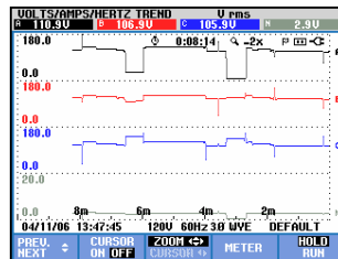
图 19-4. 趋势图显示（光标功能关闭）
