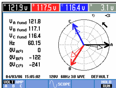
图 6-3. 正确连接的分析仪的矢量图
