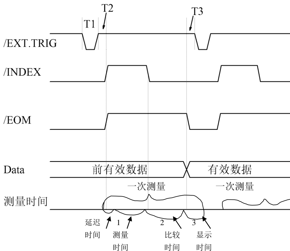
图3 时序图
