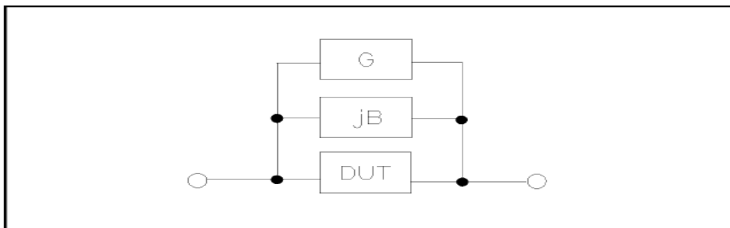
图 6-7-1 杂散导纳
