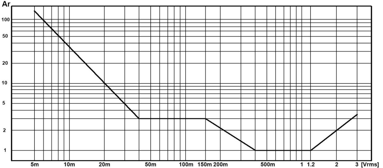
图 B 基本准确度修正曲线
