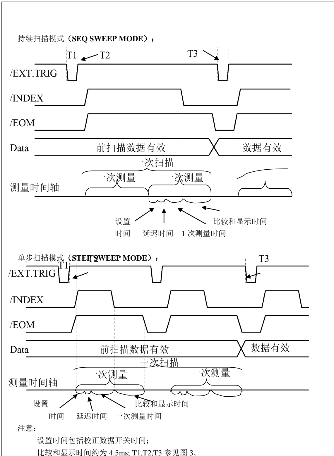
图 5 计时图解
