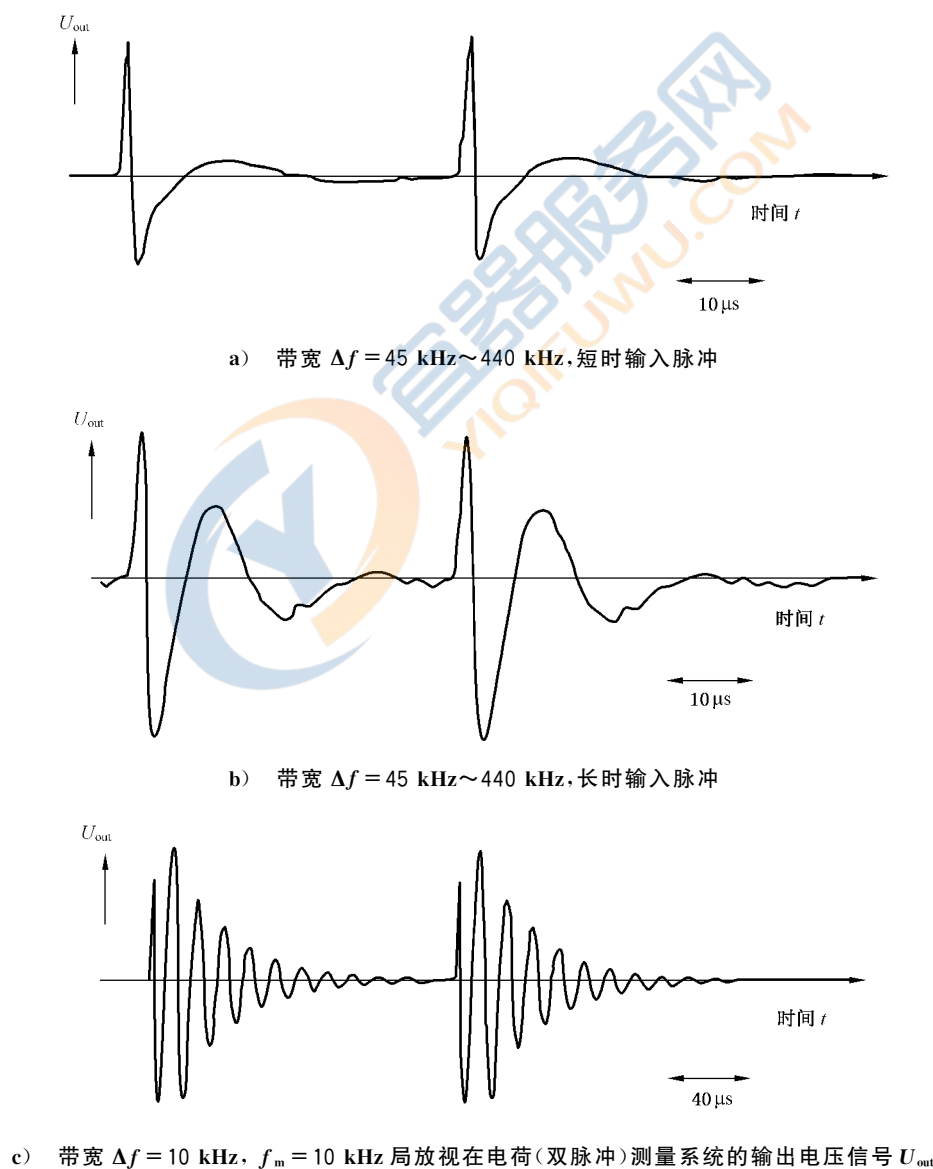
图 F.1 两种不同的局放视在电荷(双脉冲)测量系统的输出电压信号 U_{\text{out}}
