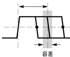
脉冲不等于宽度设置 \pm 5\% 时触发
