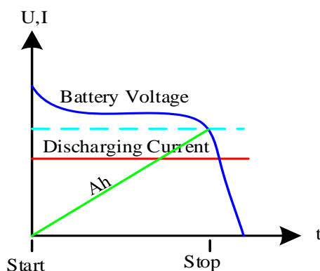
图 3-55 静态放电曲线
