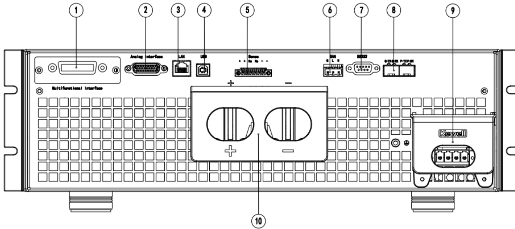
图 1-2 S7000 低压系列后面板接口一览图
