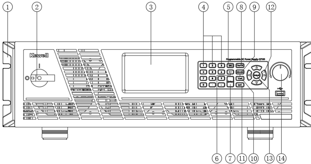
图 1-1 S7000 低压系列前面板按键与液晶屏一览表
