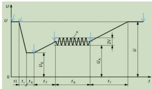
图 4-59 汽车启动波形
