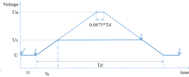
图 4-65 B 模式抛负载波形
