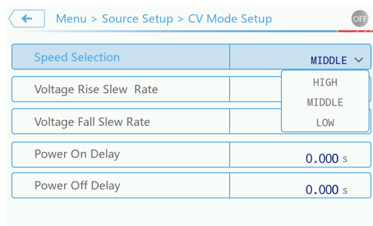
图 3-7 CV 环路选择示意图
