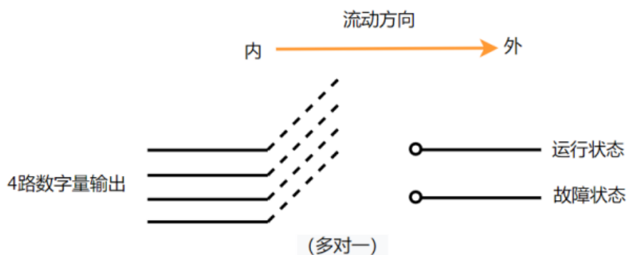
图 3-48 接口功能示意图
