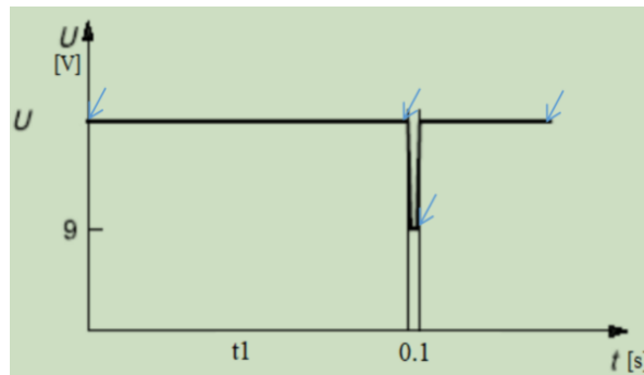
电压骤降标准波形
