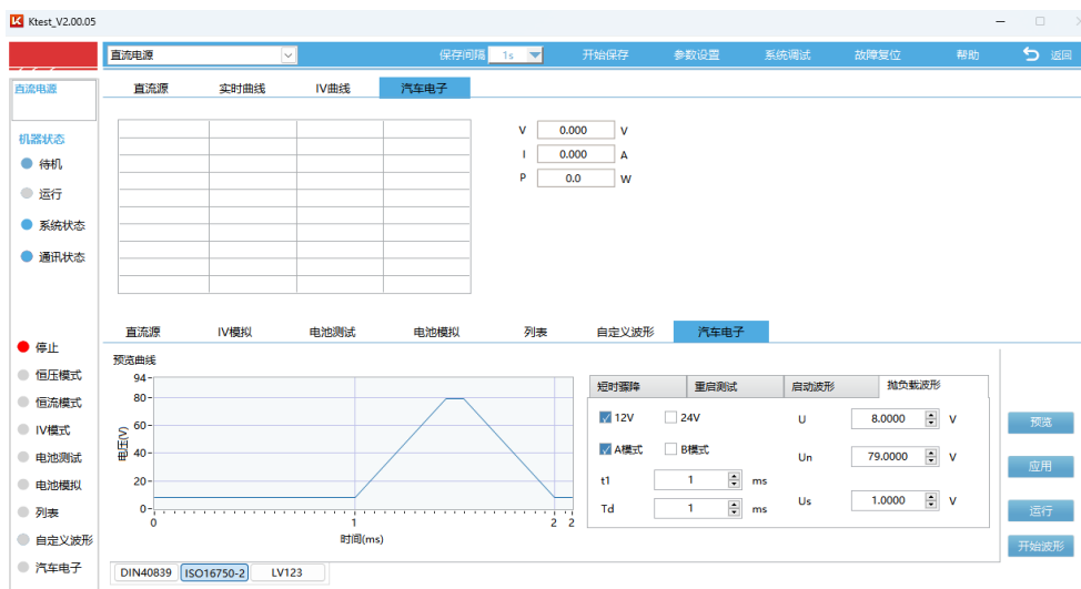
图 4-63 汽车抛负载操作界面
