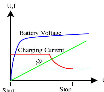
图 3-56 静态充电曲线
