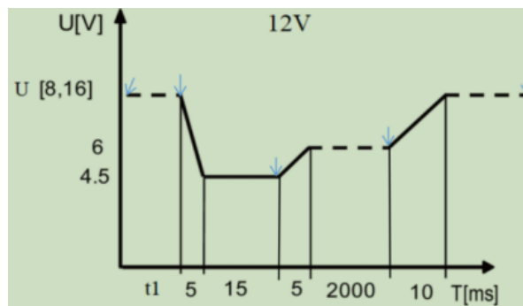
图 4-51 12V 内建标准波形
