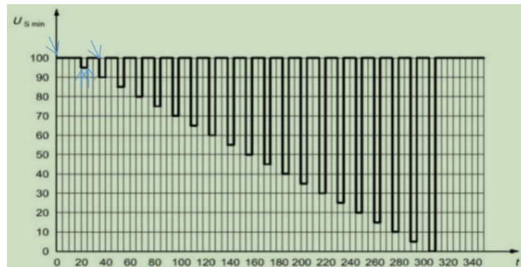
图 4-57 汽车电压重启测试波形
