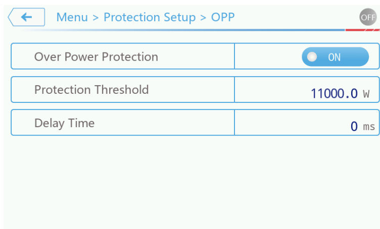
图 3-25 Over Power Protection 菜单界面示意图
