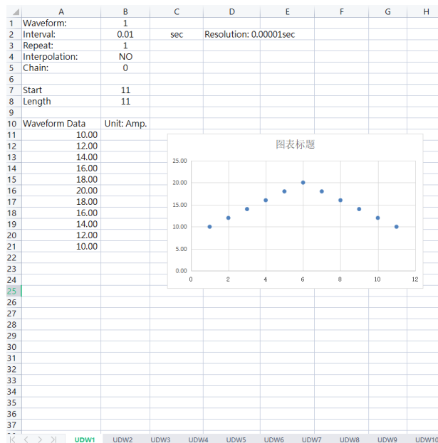
图 4-46 UDW 自定义波文档格式界面
