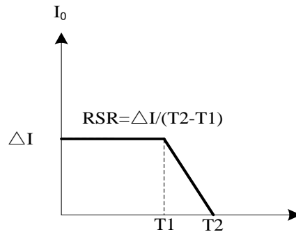
图 3-15 电流下降斜率示意图
