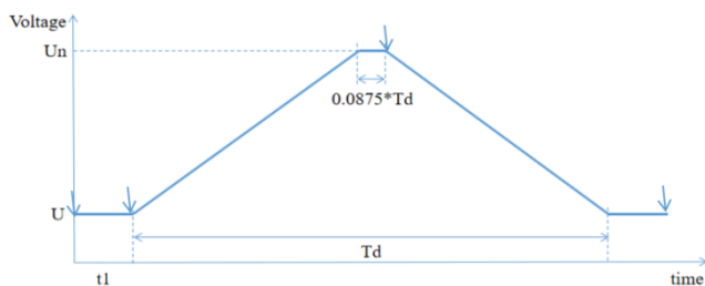
图 4-64 A 模式抛负载波形
