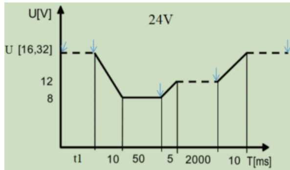
图 4-52 24V 内建标准波形
