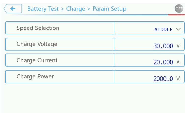
图 3-59 Charge 模式下 Parameter Setup 菜单界面示意图
