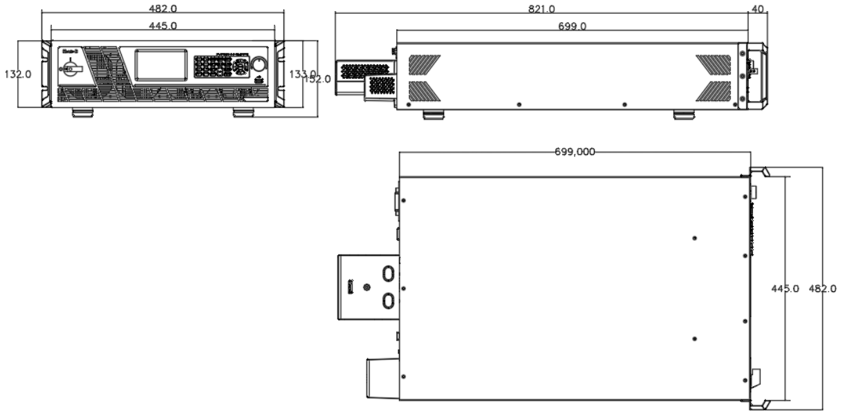
图 2-1 S7000 低压系列产品尺寸
