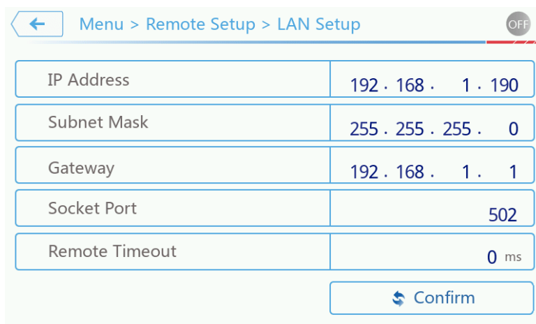
图 3-29 LAN Setup 菜单界面示意图
