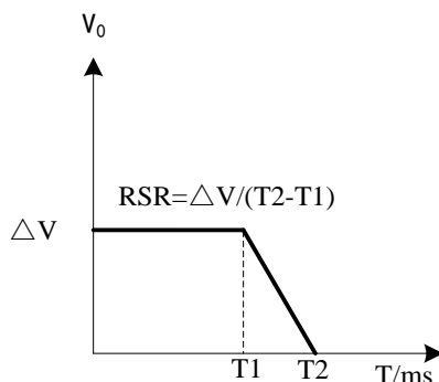
图 3-10 电压下降斜率示意图
