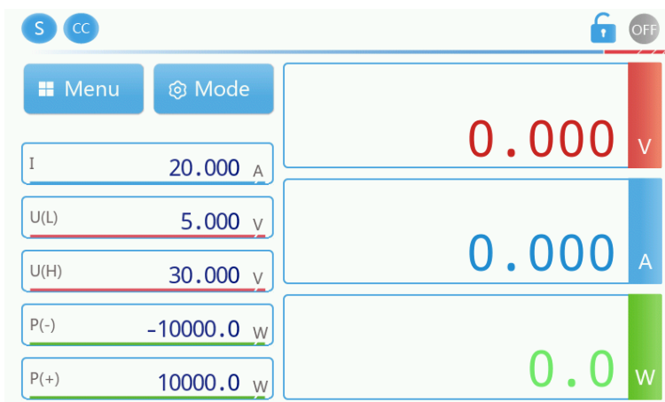
图 3-11 CC 模式下主界面示意图
