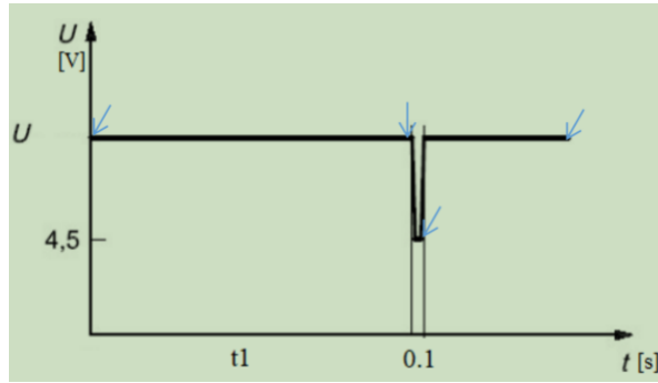
图 4-54 12V 启动短时电压骤降标准波形
