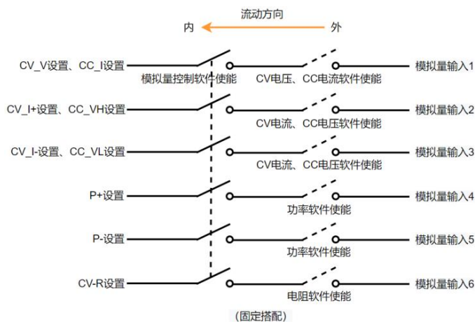
图 3-42 接口功能示意图
