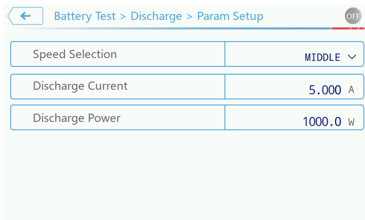
图 3-61 Parameter Setup 菜单界面示意图
