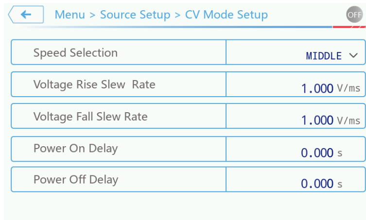
图 3-6 CV Mode Setup 菜单界面示意图
