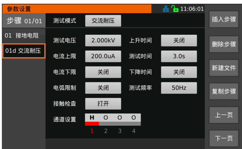
图 3-18-2 同步测试的交流耐压设置
