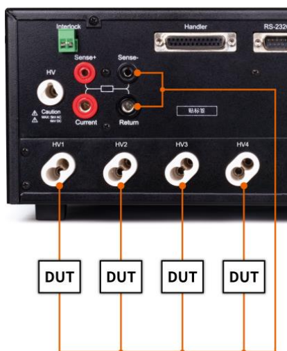
图 3-13-5 测试接线
