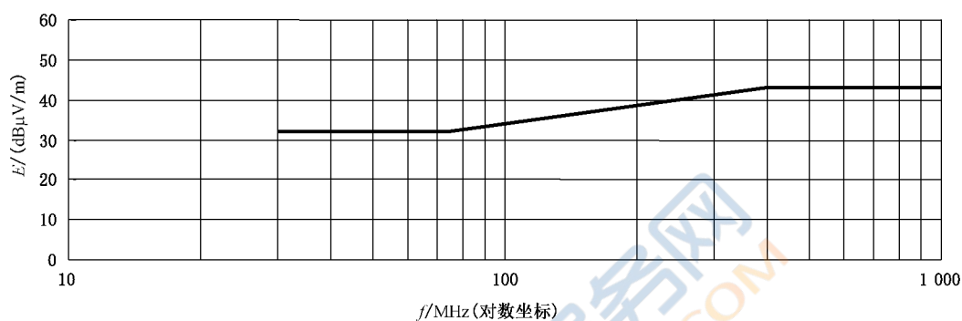
图 1 宽带电磁辐射发射限值(10 m 法)
