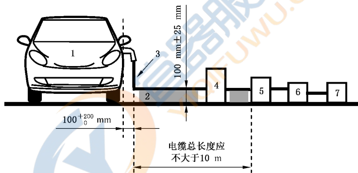
图 9 沿 AC 电源线的谐波、电压变化、波动和闪烁发射试验布置
