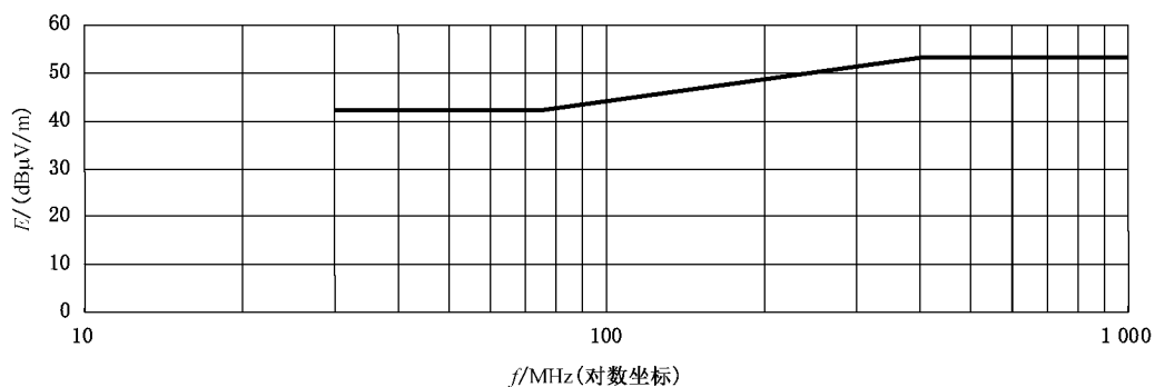
图 2 宽带电磁辐射发射限值(3 m 法)
