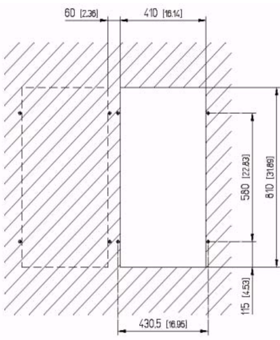
图 2-3 面板式安装
