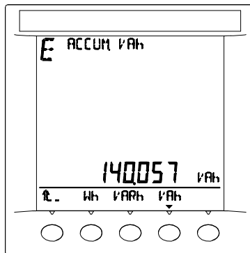
视在电能
