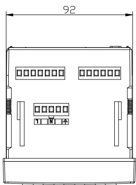
顶视图
