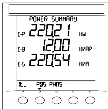
总的 PQS 值
