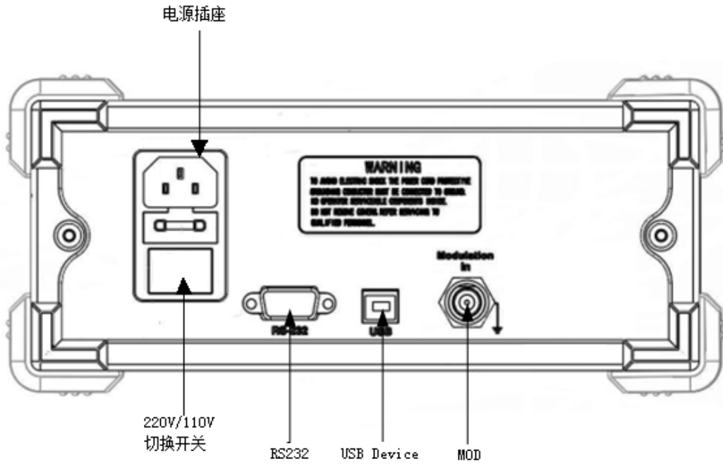
图 2-2 后面板
