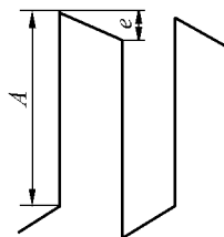
(c) 下垂检定波形
