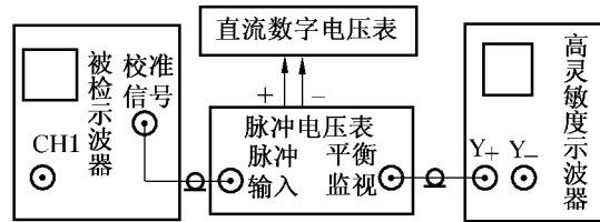
图 2 (a) 校准信号幅度检定
