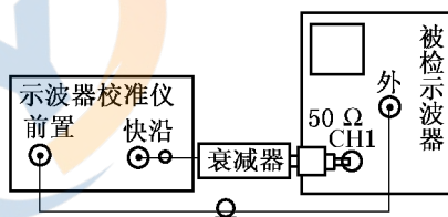
(a) 瞬间响应的检定
