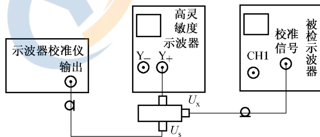
(a) 校准信号幅度检定
