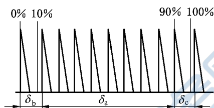
图 6 扫描线性检定波形
