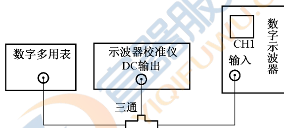
图 1 数字示波器 \Delta V 电压测量的检定
