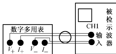
图8 输入电阻的检定
