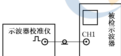
(a) 垂直偏转系数的检定
