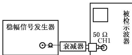
图 11 频带宽度的检定
