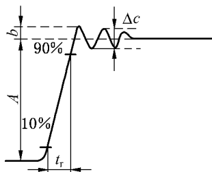
(b) 脉冲瞬态响应
