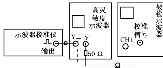
(a) 校准信号幅度检定
