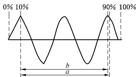
图 5 扩展扫描时间系数检定波形
