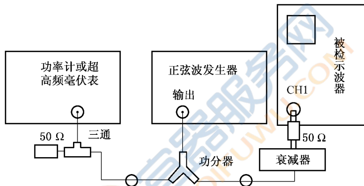
图 1 频带宽度的检定
