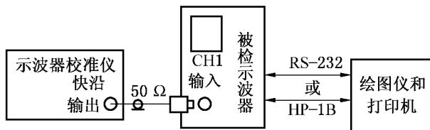
图 2 接口功能检查
