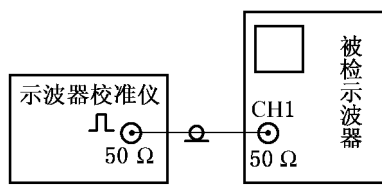
(b) 50\text{ }\Omega 垂直偏转系数的检定
