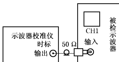
(a) 扫描时间系数的检定
