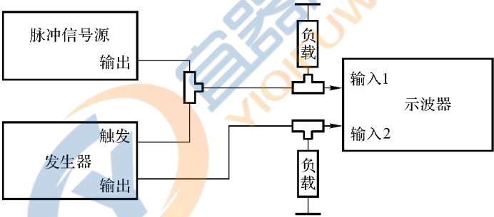
(a) 外触发延时检定
