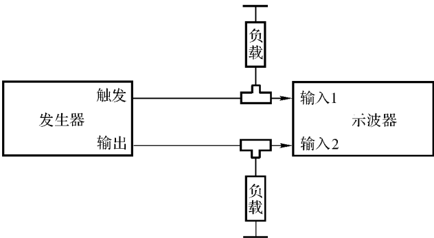
(b) 内触发延时检定
