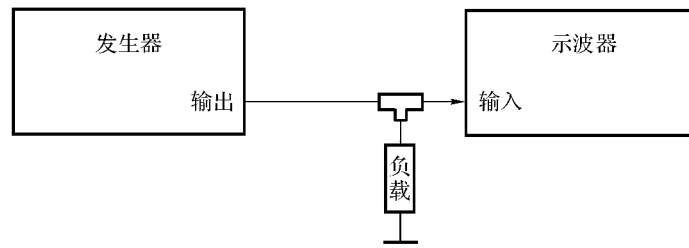
图2 脉冲幅度检定方法二
