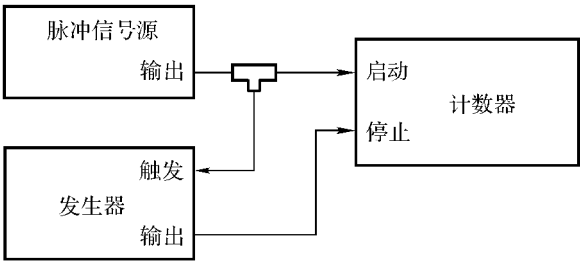
(a) 外触发延时检定
