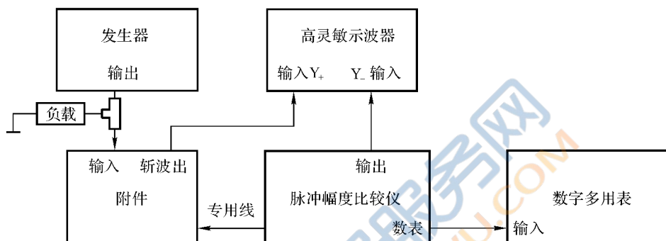
图 1 脉冲幅度检定
