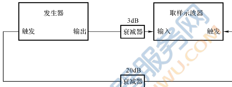
图3 脉冲上升沿检定
