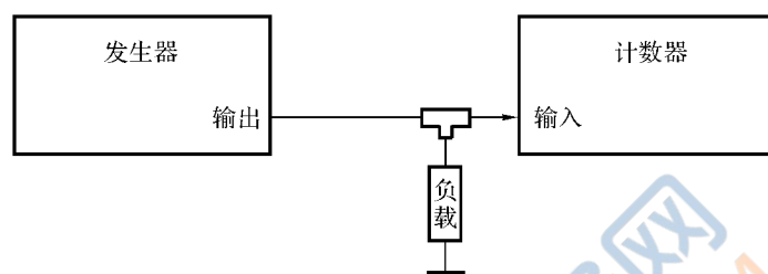
图 5 脉冲宽度及频率检定
