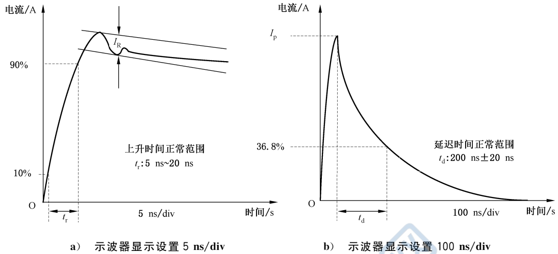
图 B.2 通过 500 Ω 电阻的电流波形
