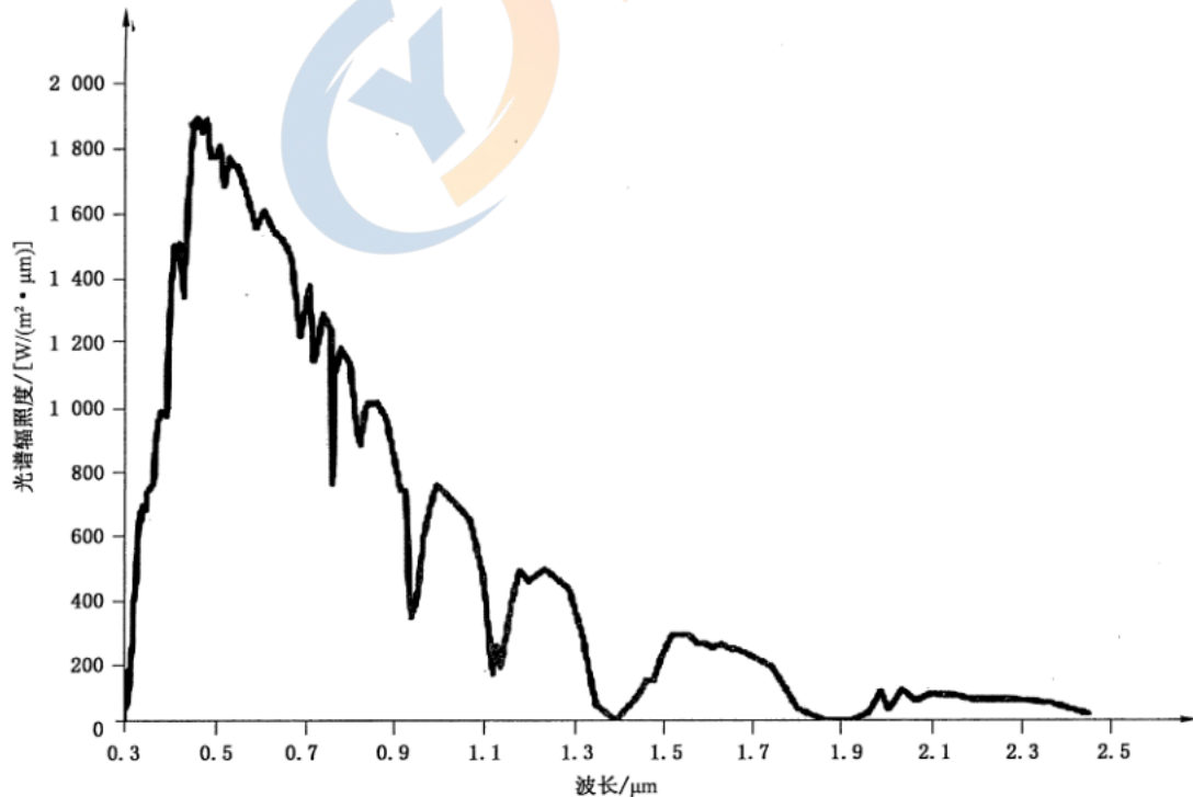
图 1 海平面的总太阳光谱辐照度
