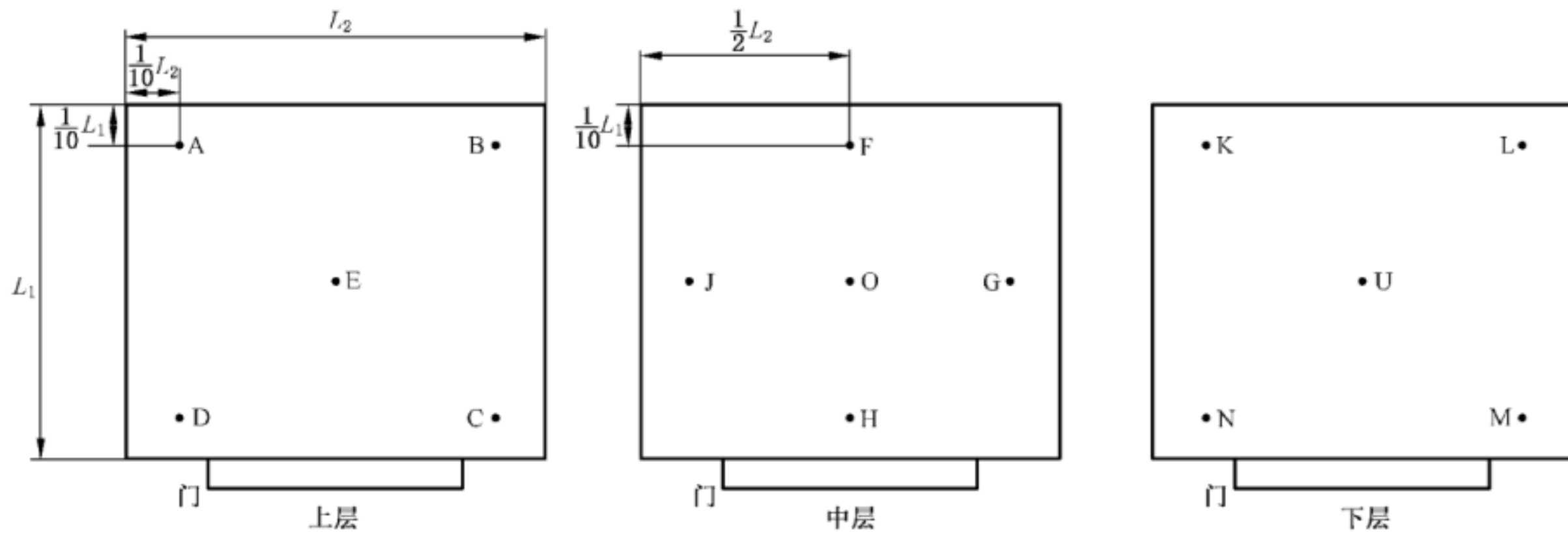
图 1 温度测量点布置位置示意图
